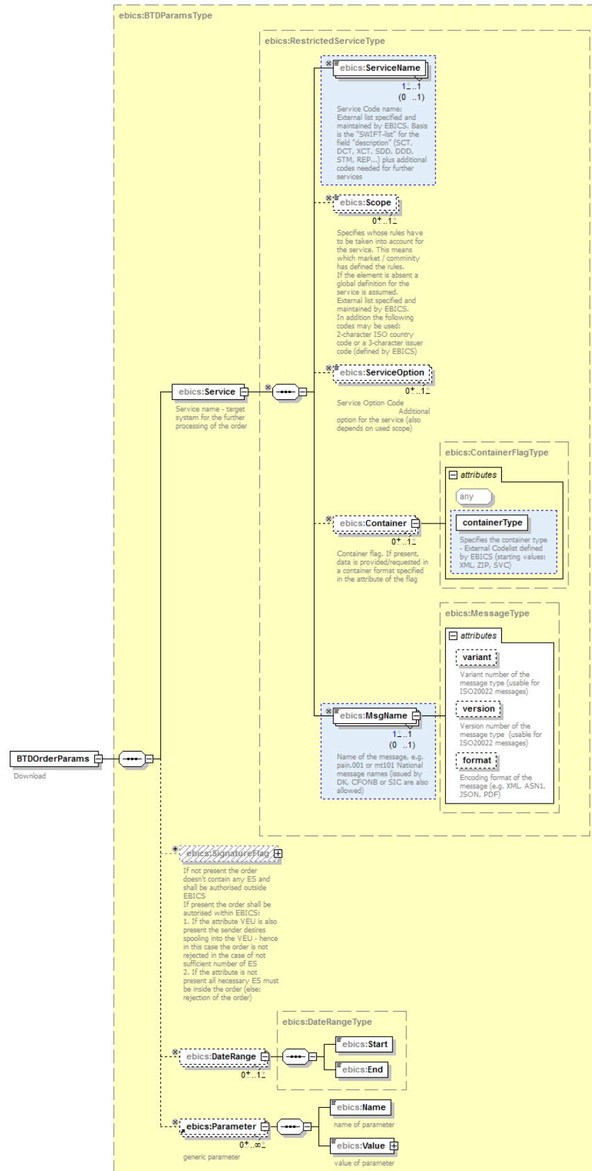
Abbildung 58: BTF-Struktur für Abholung (verwendet eingeschränkte Service-Struktur)
