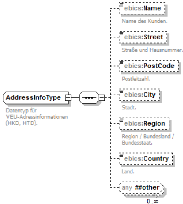
Abbildung 92: AddressInfoType (zu AddressInfo)
