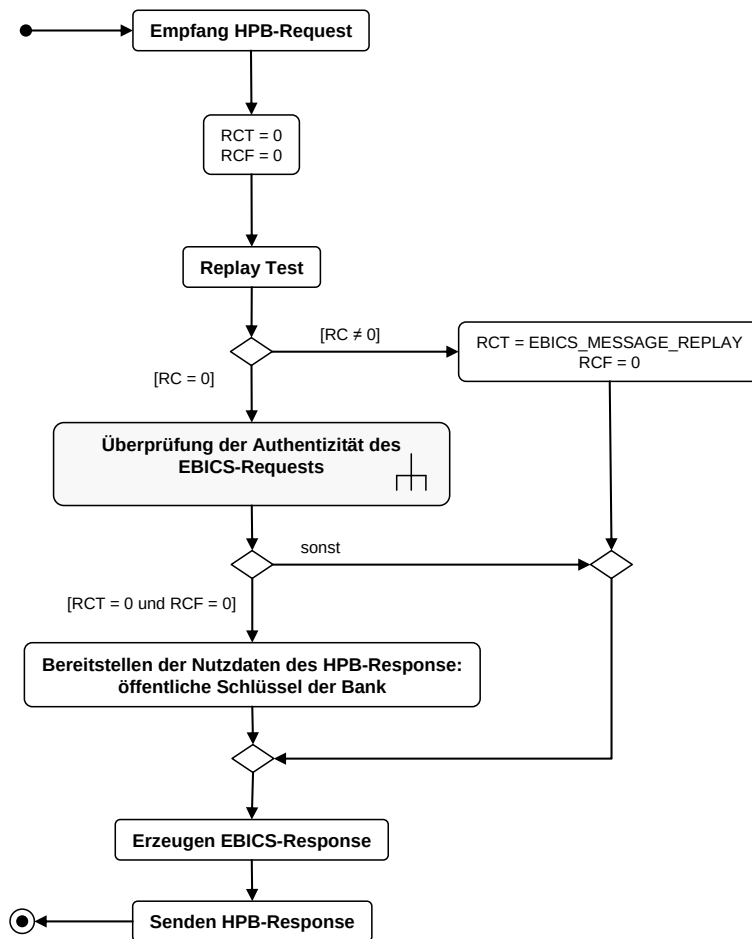
Abbildung 24: Bankseitige Verarbeitung eines HPB-Requests
