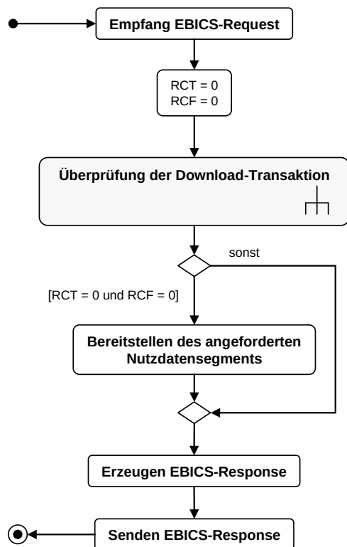
Abbildung 61: Verarbeitung eines EBICS-Requests zur Anforderung eines Nutzdatensegments
