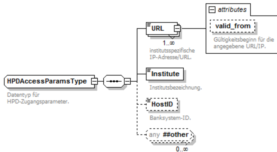
Abbildung 87: HPDAccessParamsType (zu AccessParams)
