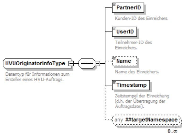
Abbildung 71: HVUOriginatorInfoType (zu OriginatorInfo)
