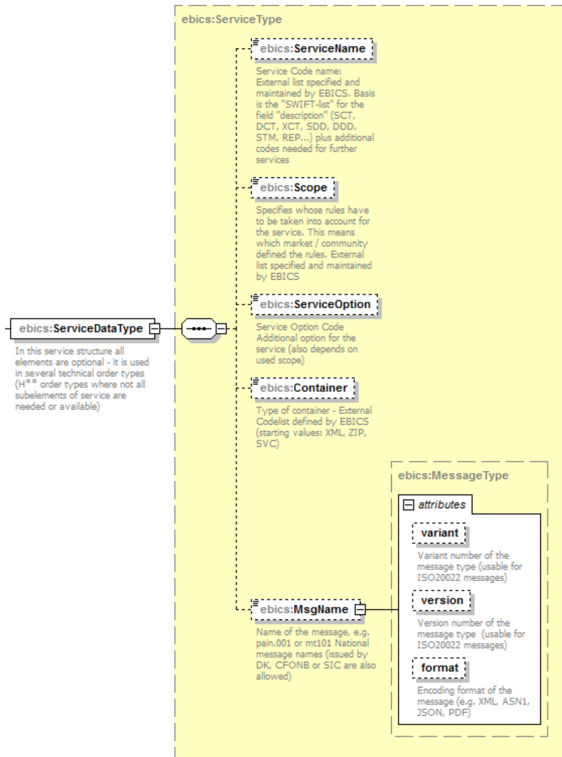
Abbildung 83: Nicht-eingeschränkte BTF-Service-Struktur nur für HVU und HVZ-Requests
