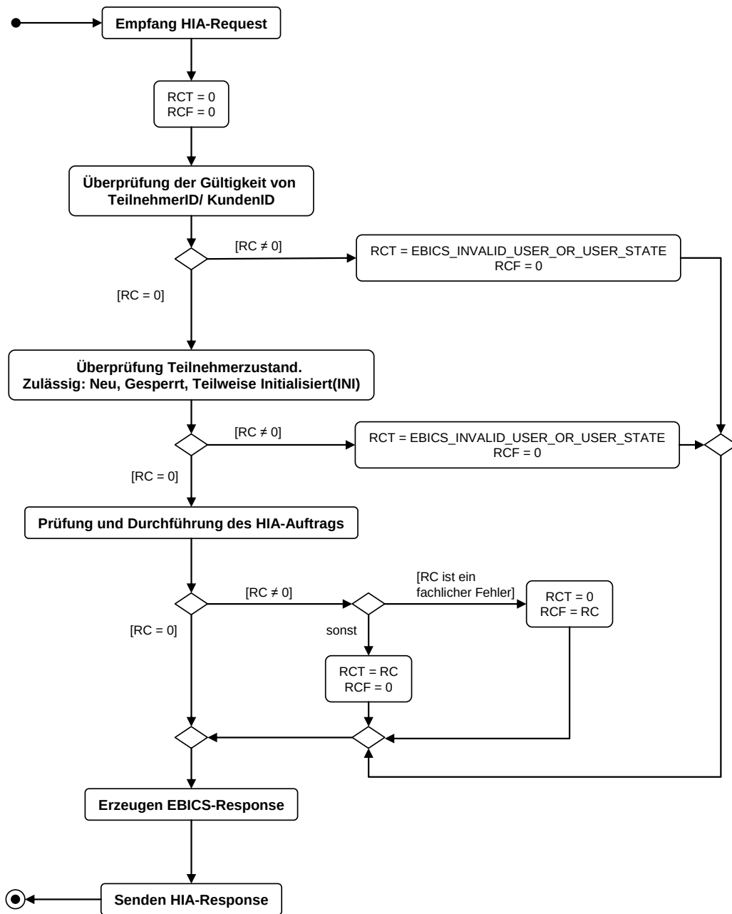
Abbildung 15: Bankseitige Verarbeitung eines HIA-Requests
