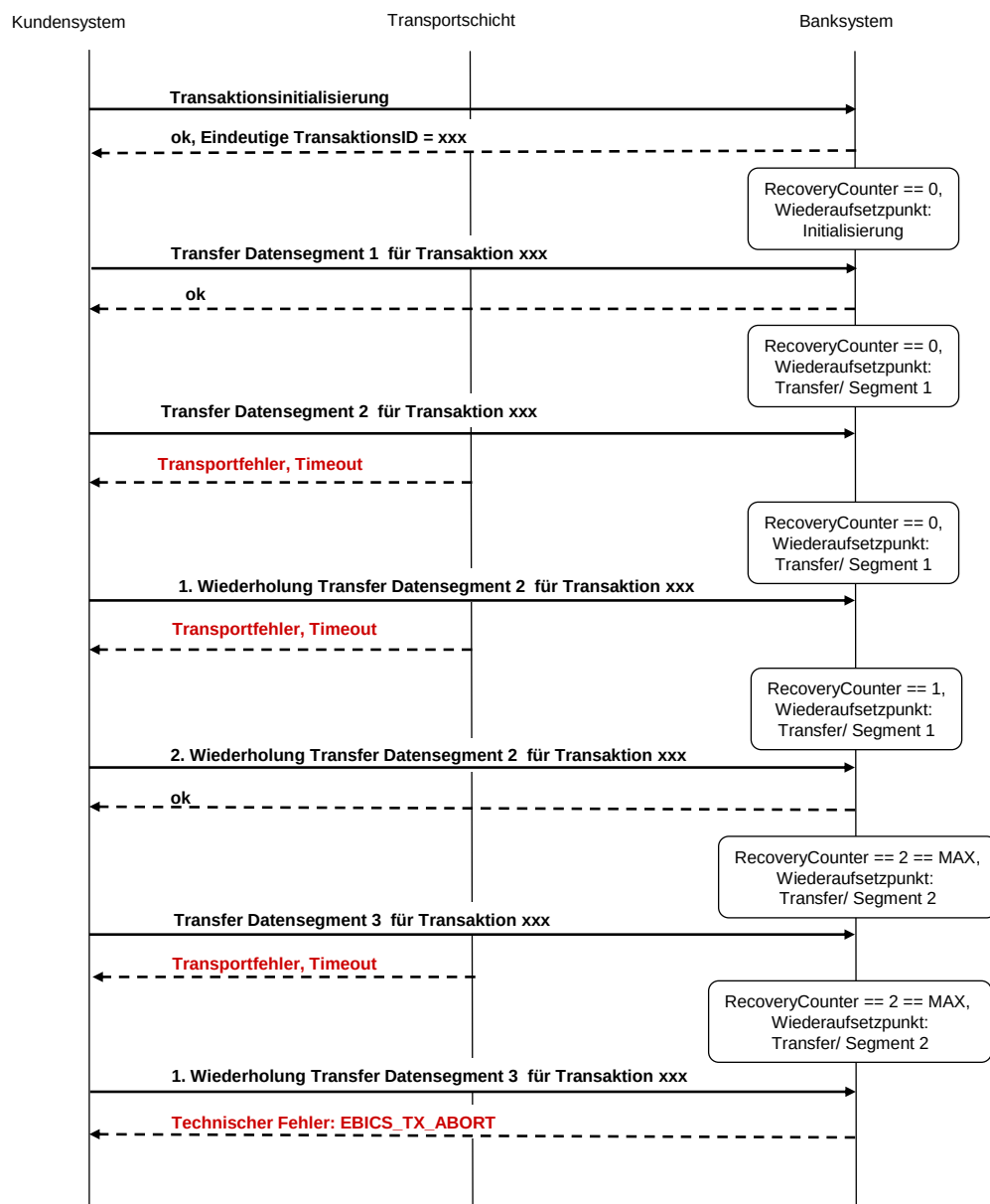
Abbildung 48: Abbruch des Recovery einer Upload-Transaktion aufgrund der Überschreitung der maximal erlaubten Zahl von Recovery-Versuchen
