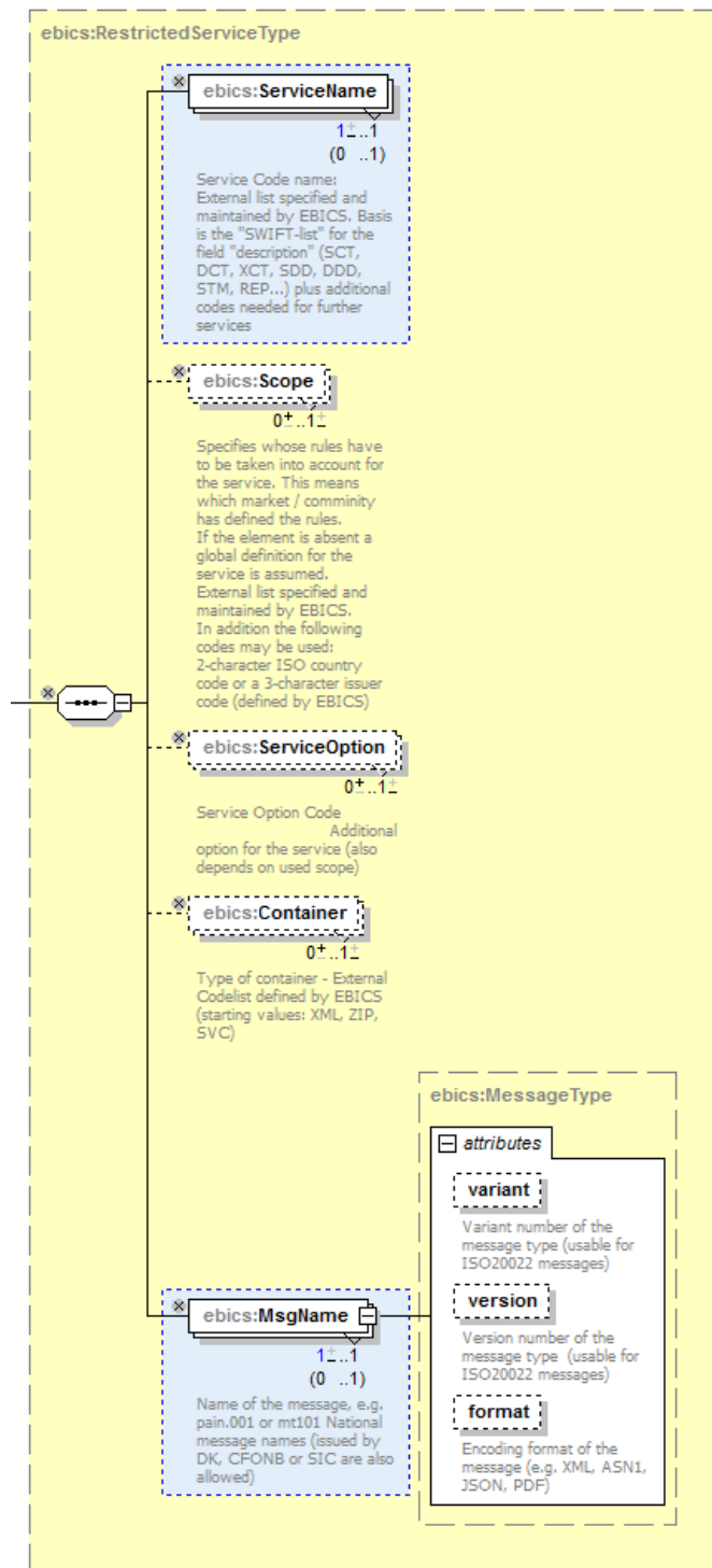
Abbildung 84: „Standard“-BTF-Servicestruktur für alle anderen Fälle
