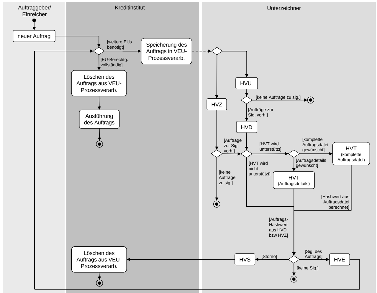
Abbildung 66: Ablaufdiagramm zur VEU
