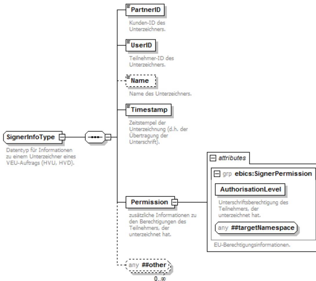
Abbildung 70: SignerInfoType (zu SignerInfo)
