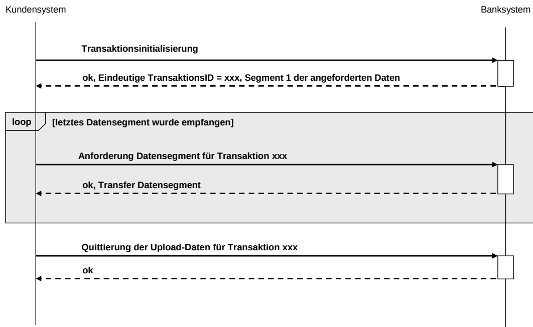
Abbildung 51: Fehlerfreier Ablauf einer Download-Transaktion
