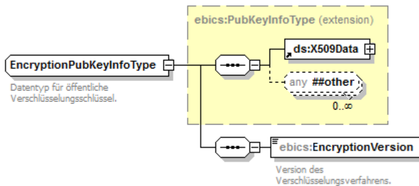
Abbildung 11: Definition des XML-Schema-Typs EncryptionPubKeyInfoType
