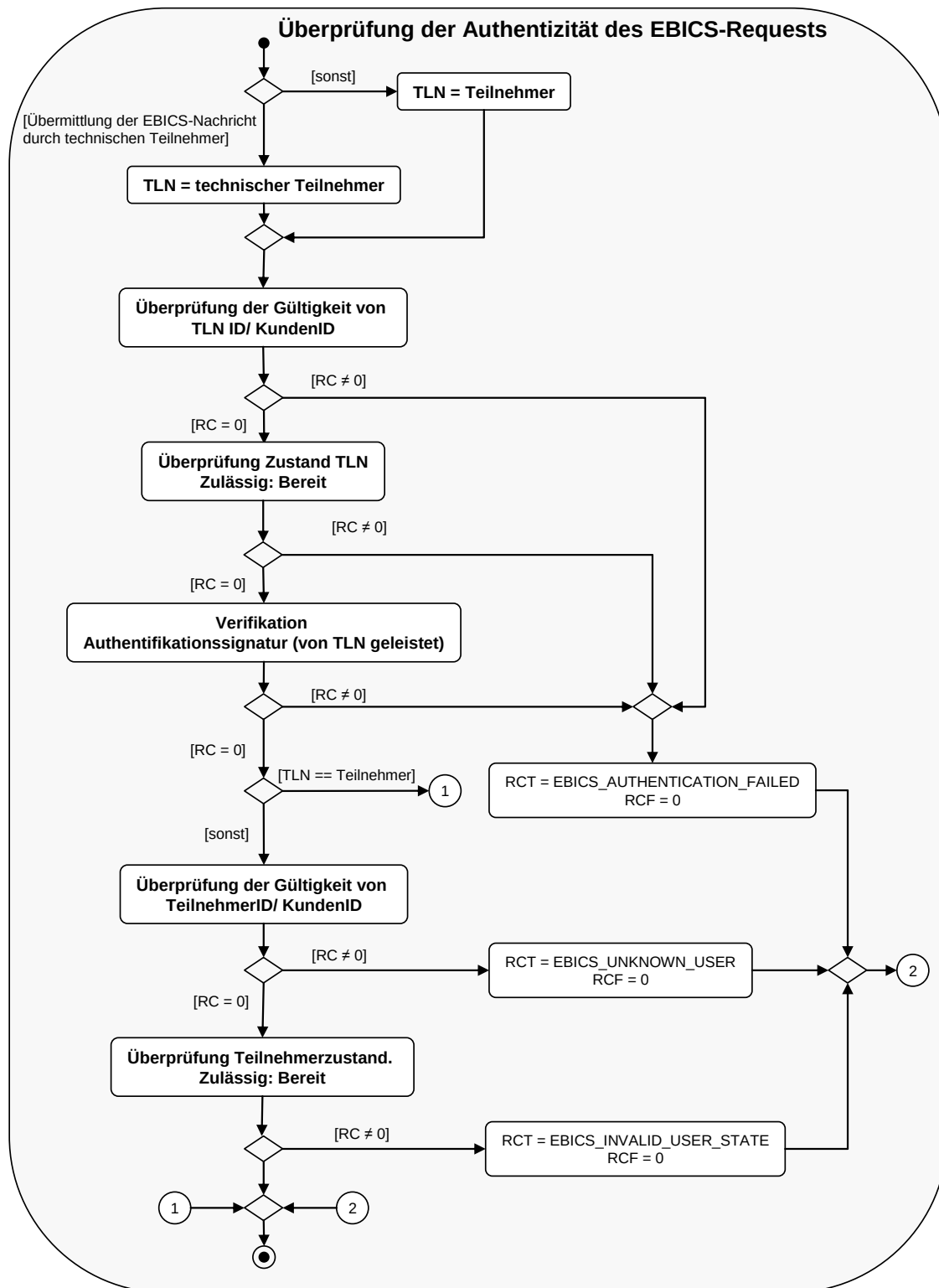
Abbildung 41: Detaillierte Beschreibung des Ablaufschritts „Überprüfung der Authentizität des EBICS-Requests“
