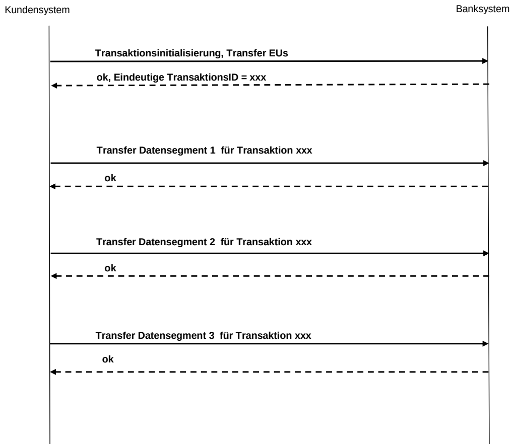
Abbildung 7: Beispielhafter Ablauf einer EBICS-Transaktion für einen Sendeauftrag
