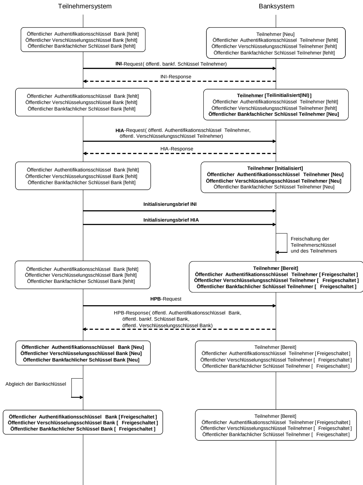
Abbildung 13: Beispielhafter Ablauf: Teilnehmerinitialisierung mit anschließender Abholung und Überprüfung der Bankschlüssel (wenn mit INI/HIA initialisiert wird)
