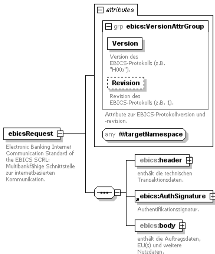
Abbildung 3: Wurzelstruktur des EBICS-Protokolls
