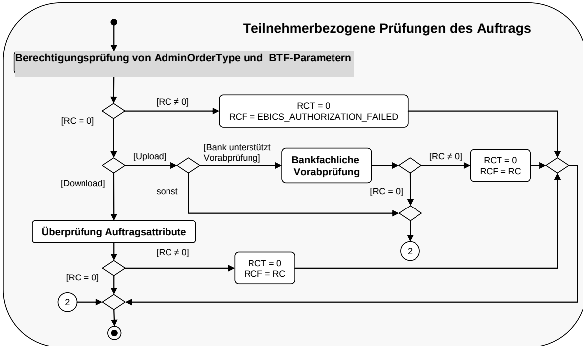
Abbildung 42: Detaillierte Beschreibung des Ablaufschritts „Teilnehmerbezogene Prüfungen des Auftrags“
