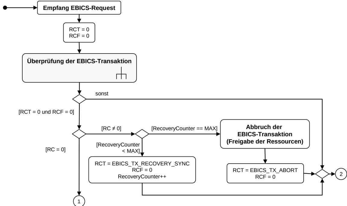
Abbildung 46: Verarbeitung eines EBICS-Requests zur Übermittlung eines Nutzdatensegments (1. Teil)
