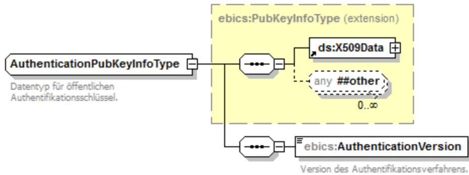
Abbildung 9: Definition des XML-Schema-Typs AuthenticationPubKeyInfoType
