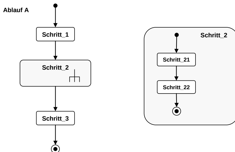
Abbildung 2 Verschachtelung von Aktivitäten
