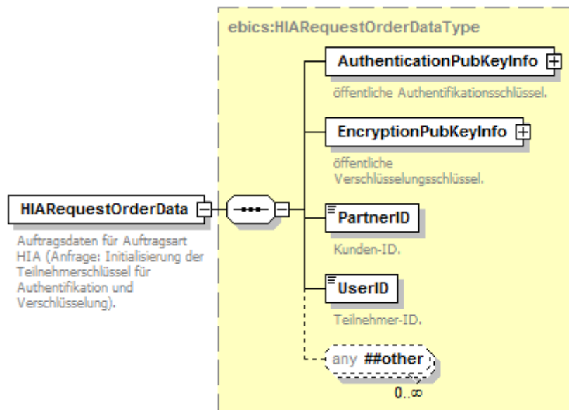
Abbildung 18: Definition des XML-Schema-Elements HIRequestOrderData der Auftragsdaten für HIA
