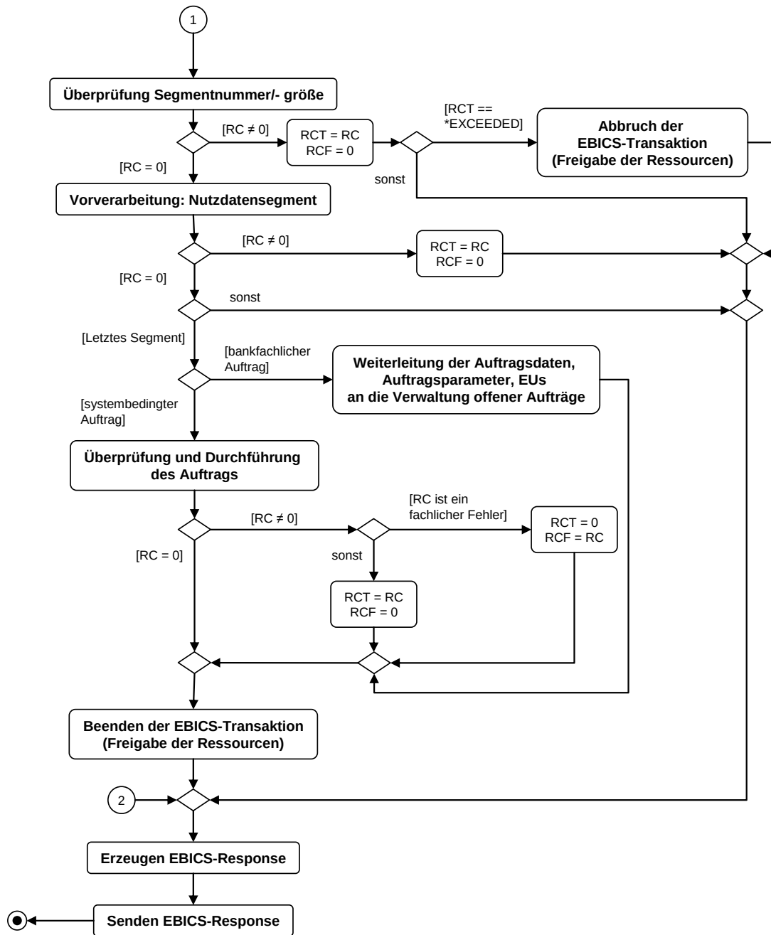
Abbildung 47: Verarbeitung eines EBICS-Requests zur Übermittlung eines Nutzdatensegments (2. Teil)
