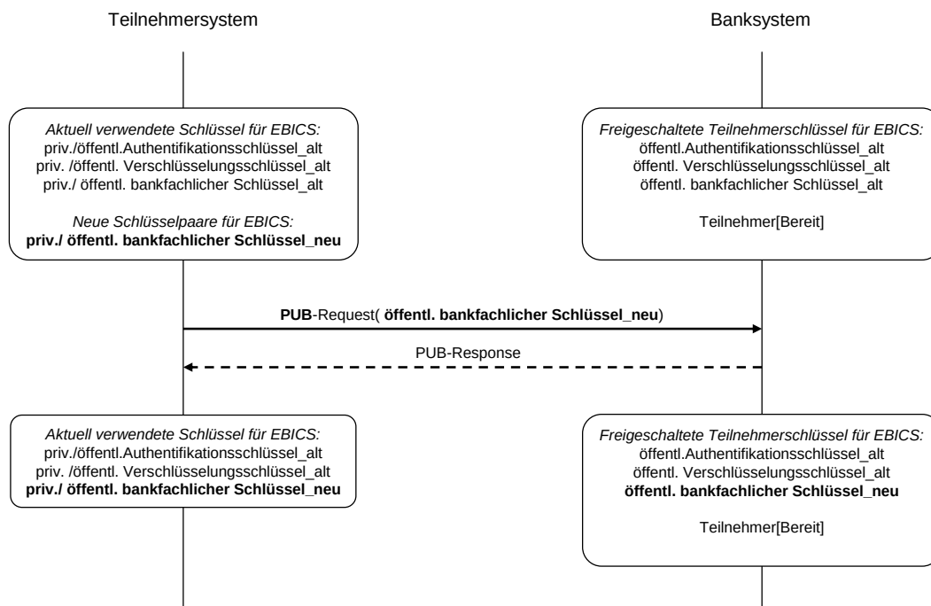
Abbildung 28: Änderung des bankfachlichen Teilnehmerschlüssels mittels PUB
