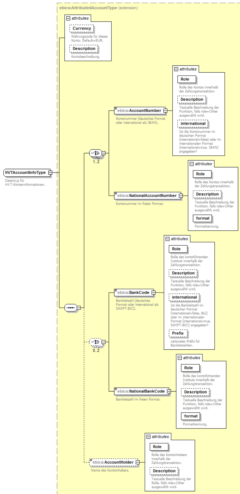
Abbildung 80: HVTAccountInfoType (zu AccountInfo)
