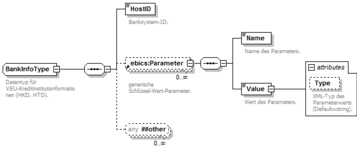
Abbildung 93: BankInfoType (zu BankInfo)
