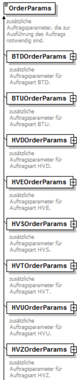
Abbildung 6: OrderParams
