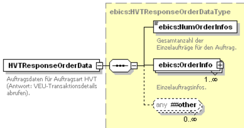
Abbildung 78: HVTResponseOrderData
