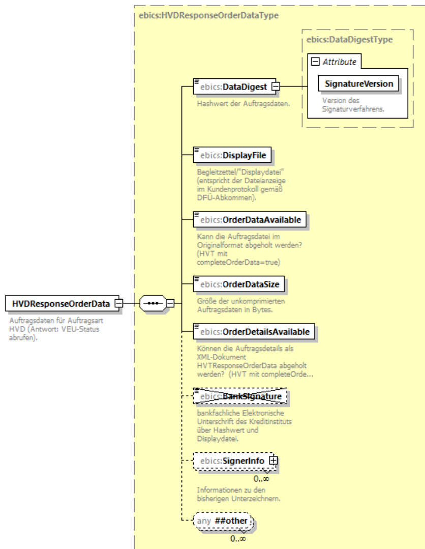
Abbildung 76: HVDResponseOrderData
