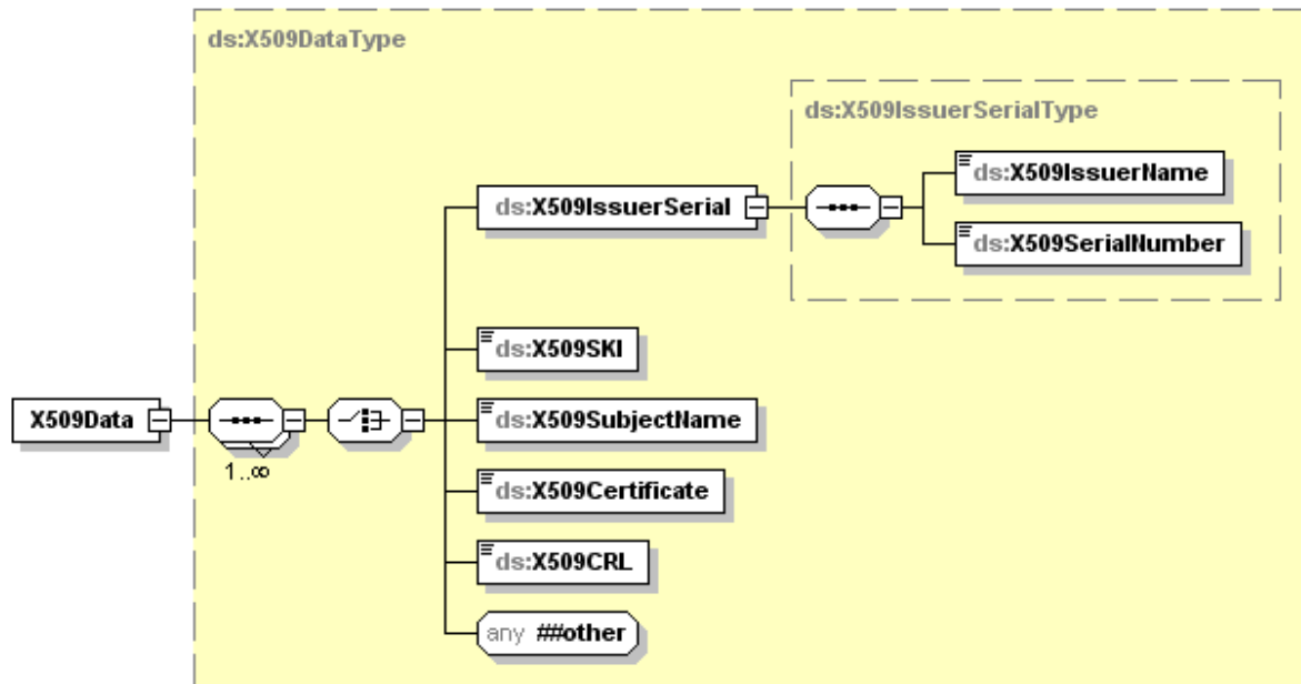
Abbildung 5: X509DataType
