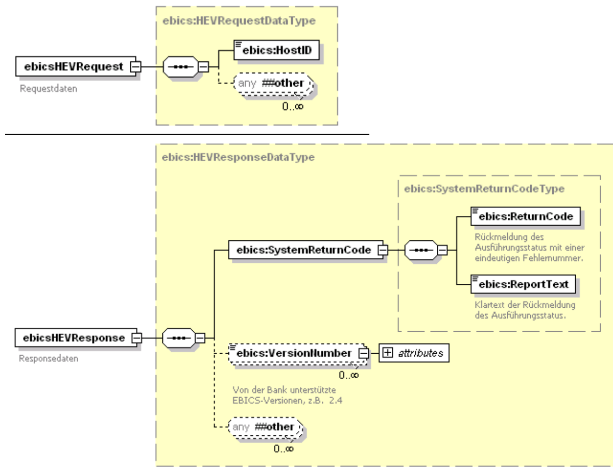
Abbildung 98: HEVRequest / HEVResponse
