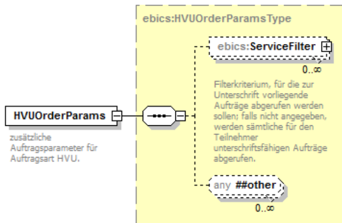
Abbildung 67: HVUOrderParams
