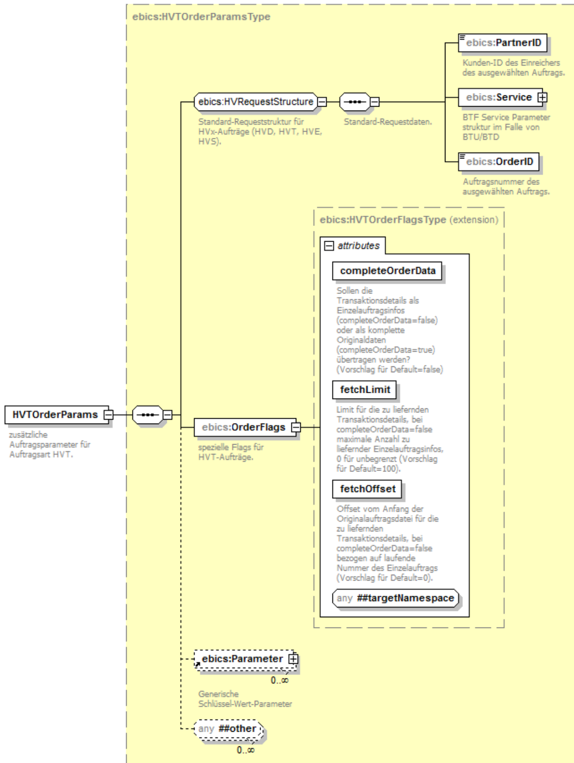
Abbildung 77: HVTOrderParams
