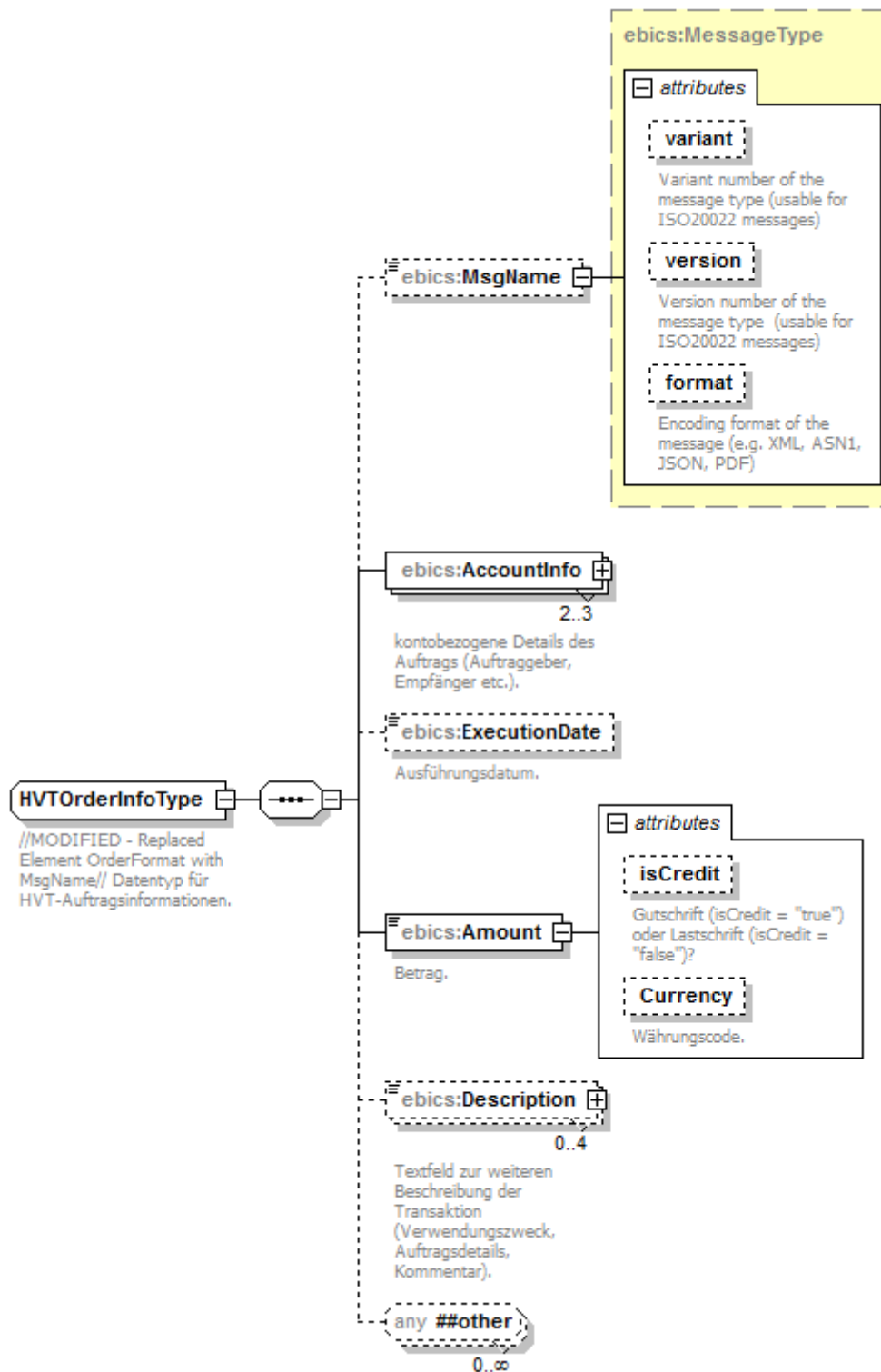
Abbildung 79: HVTOrderInfoType (zu OrderInfo)
