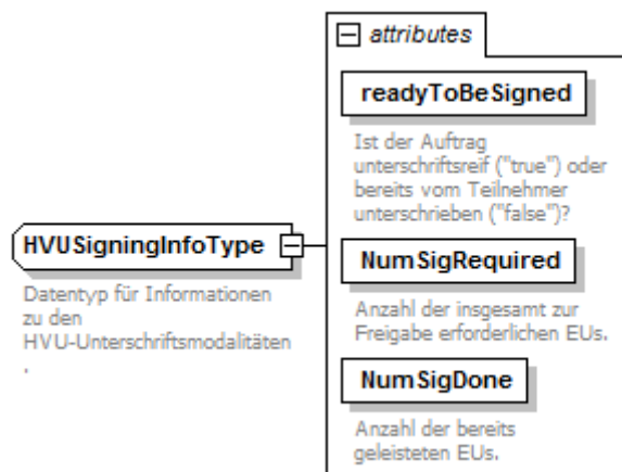
Abbildung 69: HVUSigningInfoType (zu SigningInfo)
