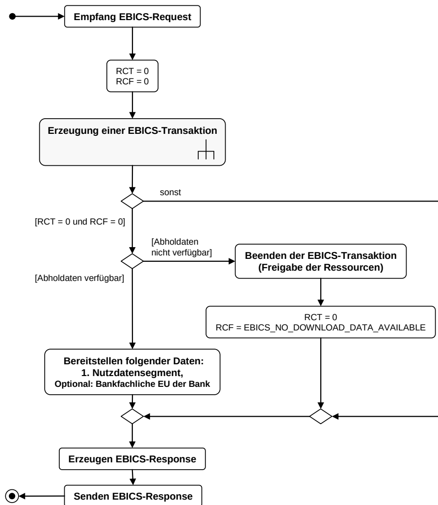
Abbildung 59: Verarbeitung des EBICS-Requests der Initialisierungsphase einer Download-Transaktion
