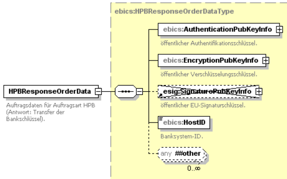
Abbildung 25: Definition des XML-Schema-Elements HPBResponseOrderData der Auftragsdaten für HPB
