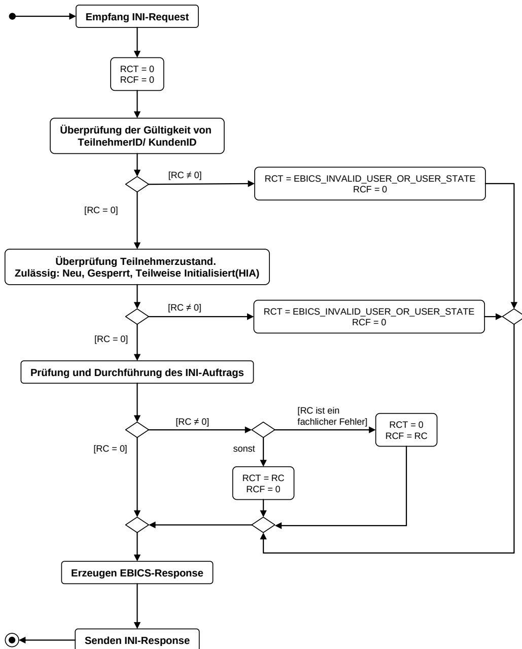
Abbildung 14: Bankseitige Verarbeitung eines INI-Requests
