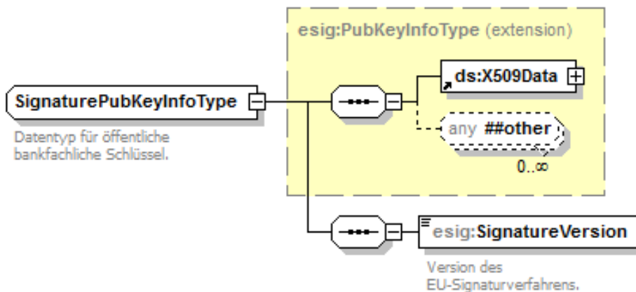
Abbildung 10: Definition des XML-Schema-Typs SignaturePubKeyInfoType
