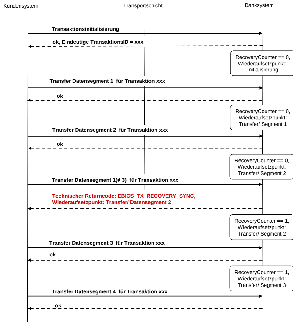
Abbildung 49: Recovery einer Upload-Transaktion mit expliziter Synchronisation zwischen Kunden- und Banksystem
