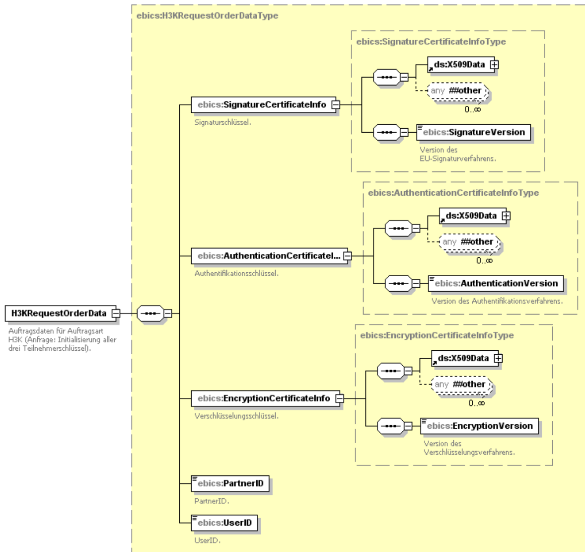
Abbildung 23: Definition des XML-Schema-Elements H3KRequestOrderData für H3KOrder Data
