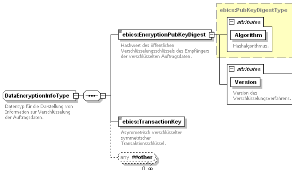
Abbildung 99: Definition des XML-Schema Typs DataEncryptionInfoType
