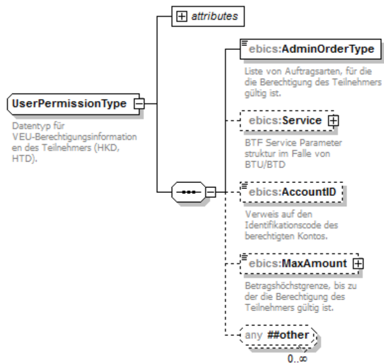
Abbildung 96: UserPermissionType (zu Permission)
