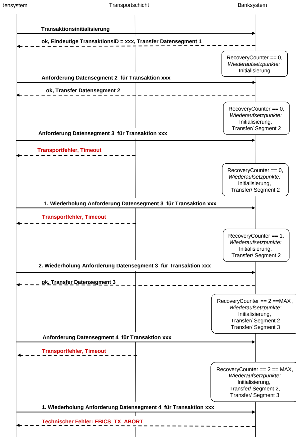
Abbildung 63: Abbruch des Recovery einer Download-Transaktion aufgrund der Überschreitung der maximal erlaubten Zahl von Recovery-Versuchen
