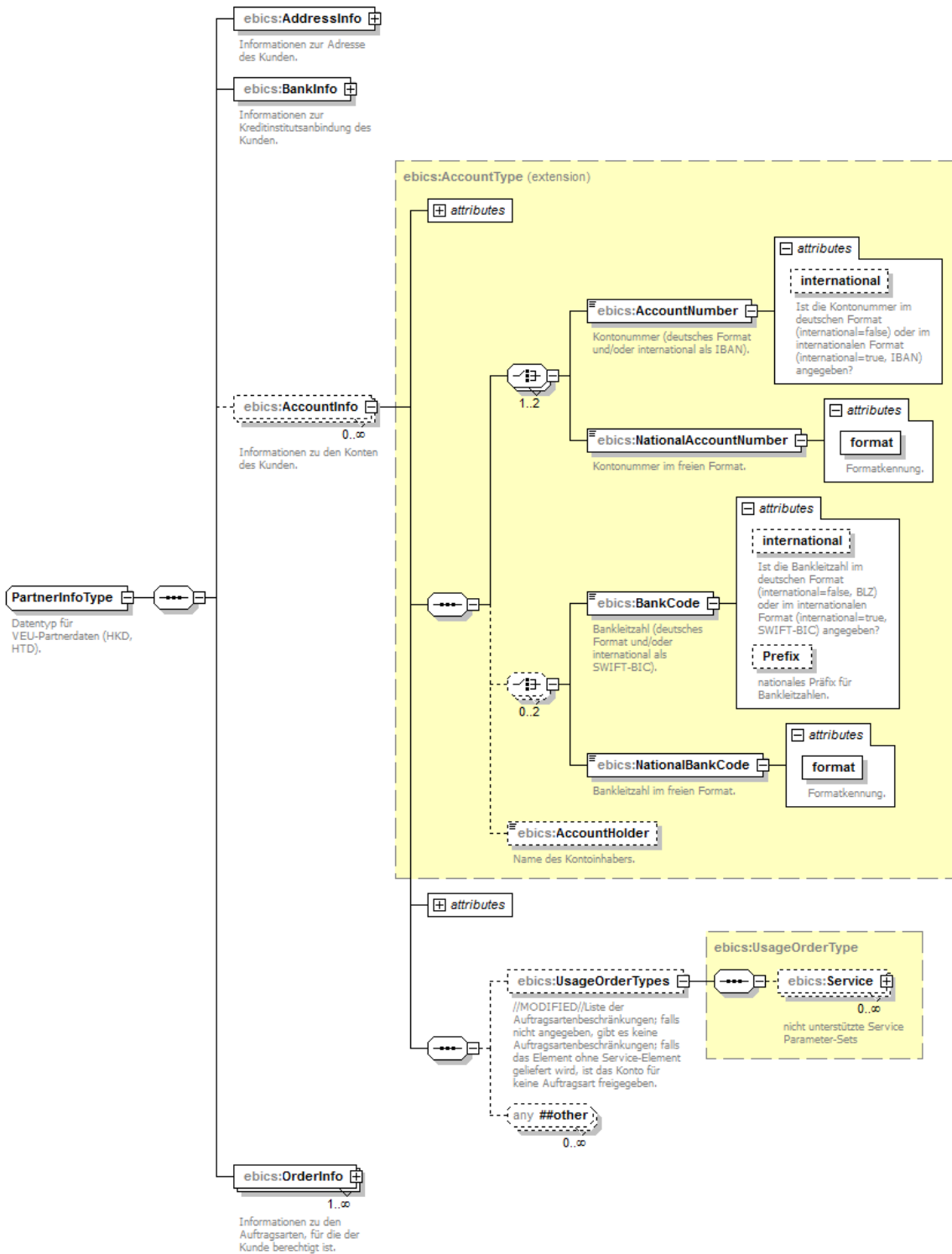
Abbildung 91: PartnerInfoType (zu PartnerInfo)
