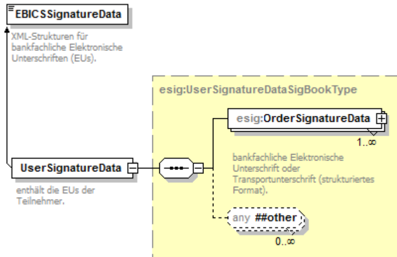
Abbildung 4: XML-Strukturen UserSignatureData für die EUs eines Auftrags (in strukturierter Form)
