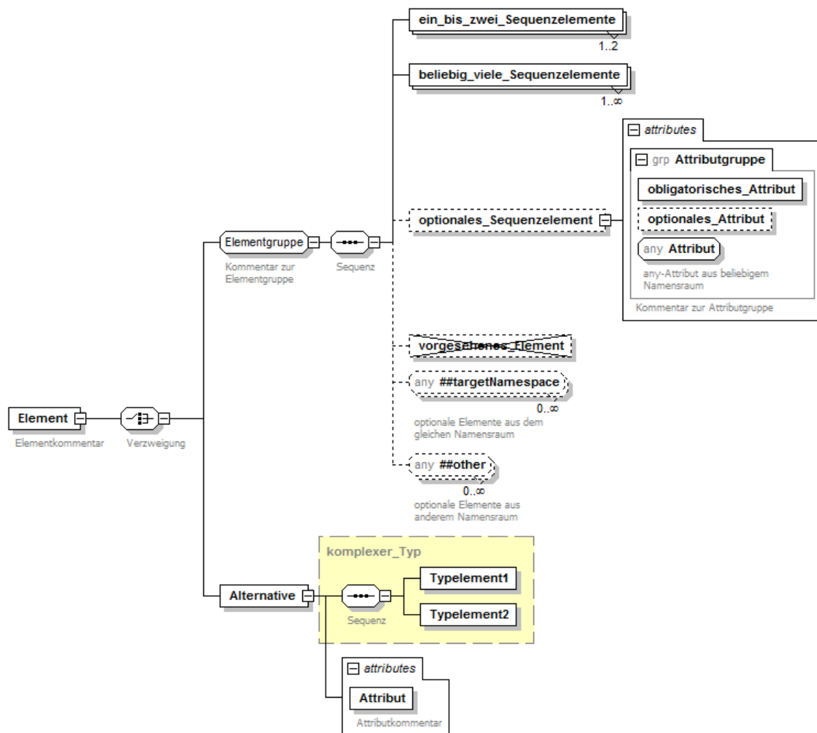
Abbildung 1: Symbolik für XML-Schema
