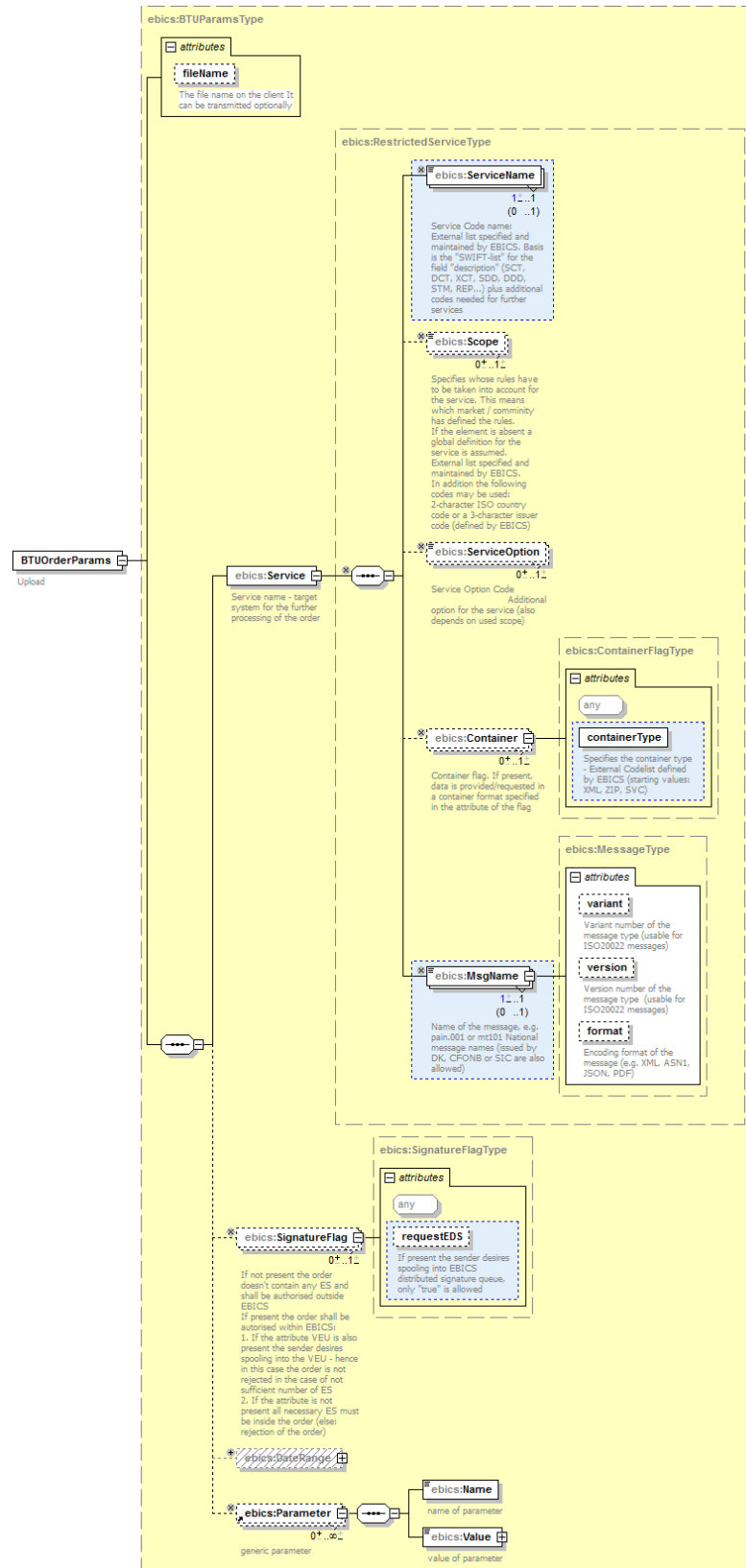
Abbildung 40: BTF-Struktur für Senden (verwendet eingeschränkte Service-Struktur)
