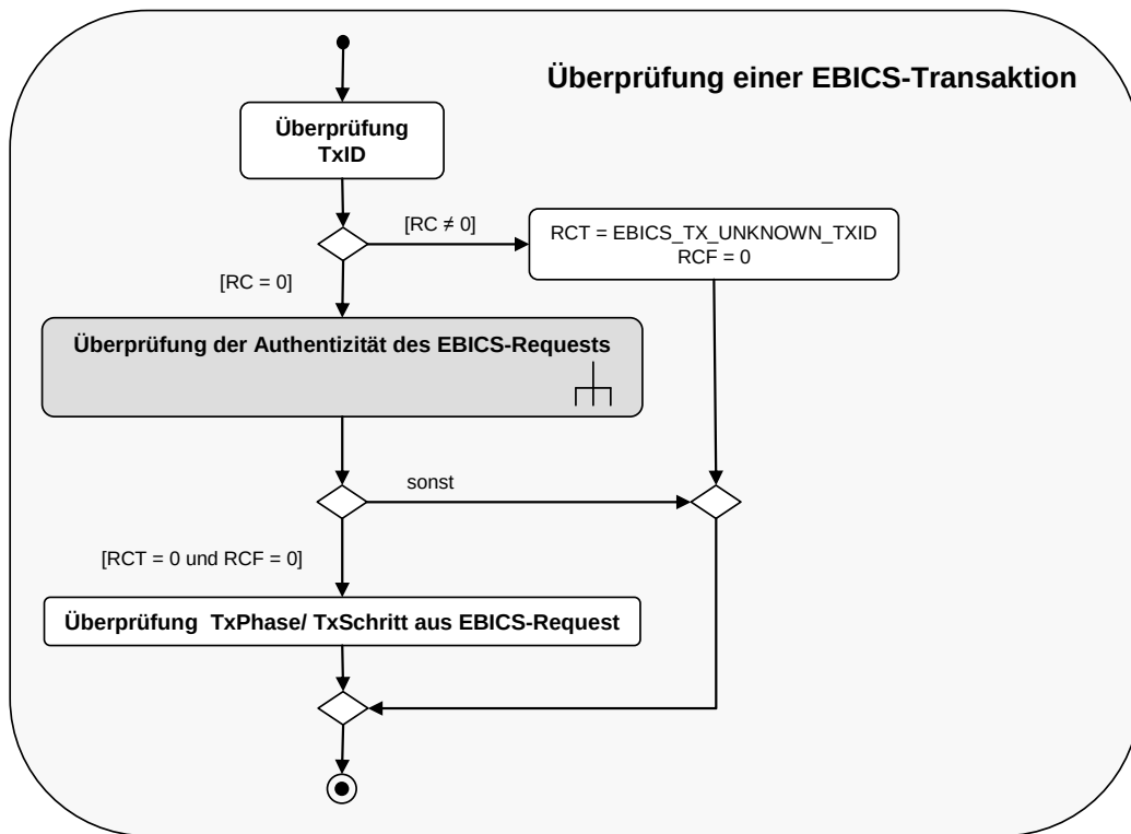
Abbildung 45: Detaillierte Beschreibung des Ablaufschritts „Überprüfung einer EBICS-Transaktion“
