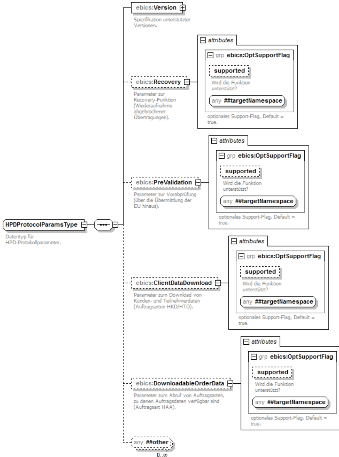
Abbildung 88: HPDProtocolParamsType (zu ProtocolParams)
