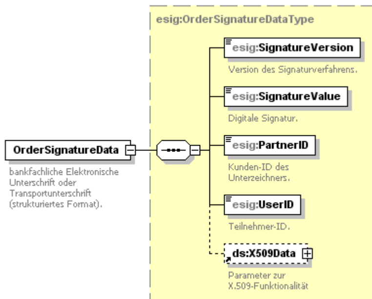
Abbildung 100: OrderSignatureData – strukturierte Elektronische Unterschrift
