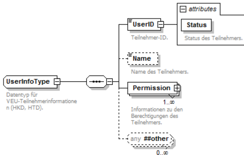
Abbildung 95: UserInfoType (zu UserInfo)
