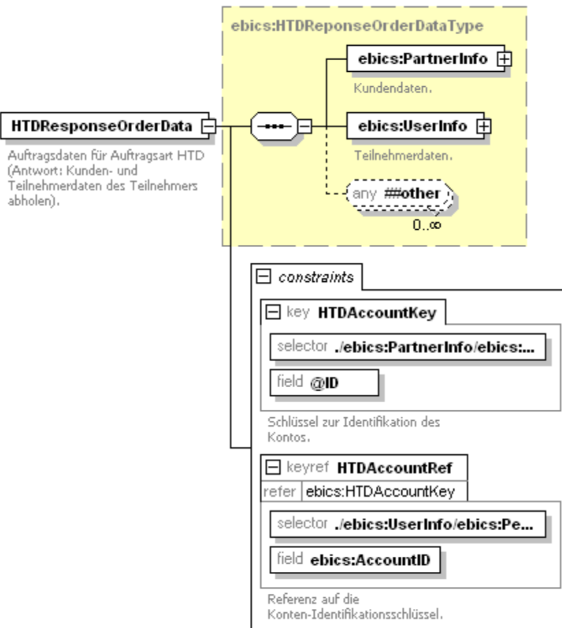
Abbildung 97: HTDResponseOrderData
