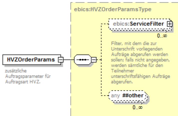
Abbildung: 72 HVZOrderParams
