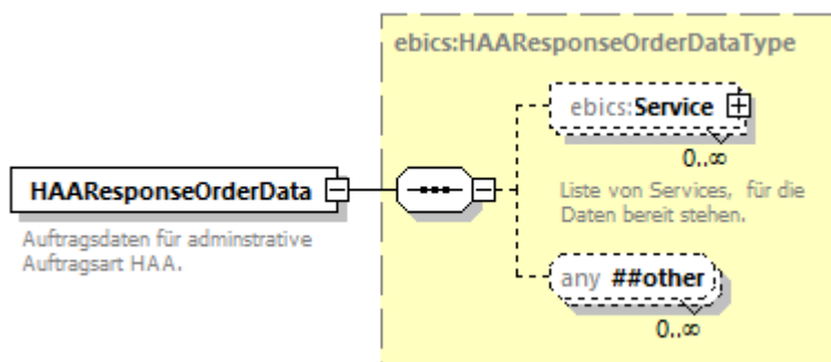
Abbildung 85: HAAResponseOrderData
