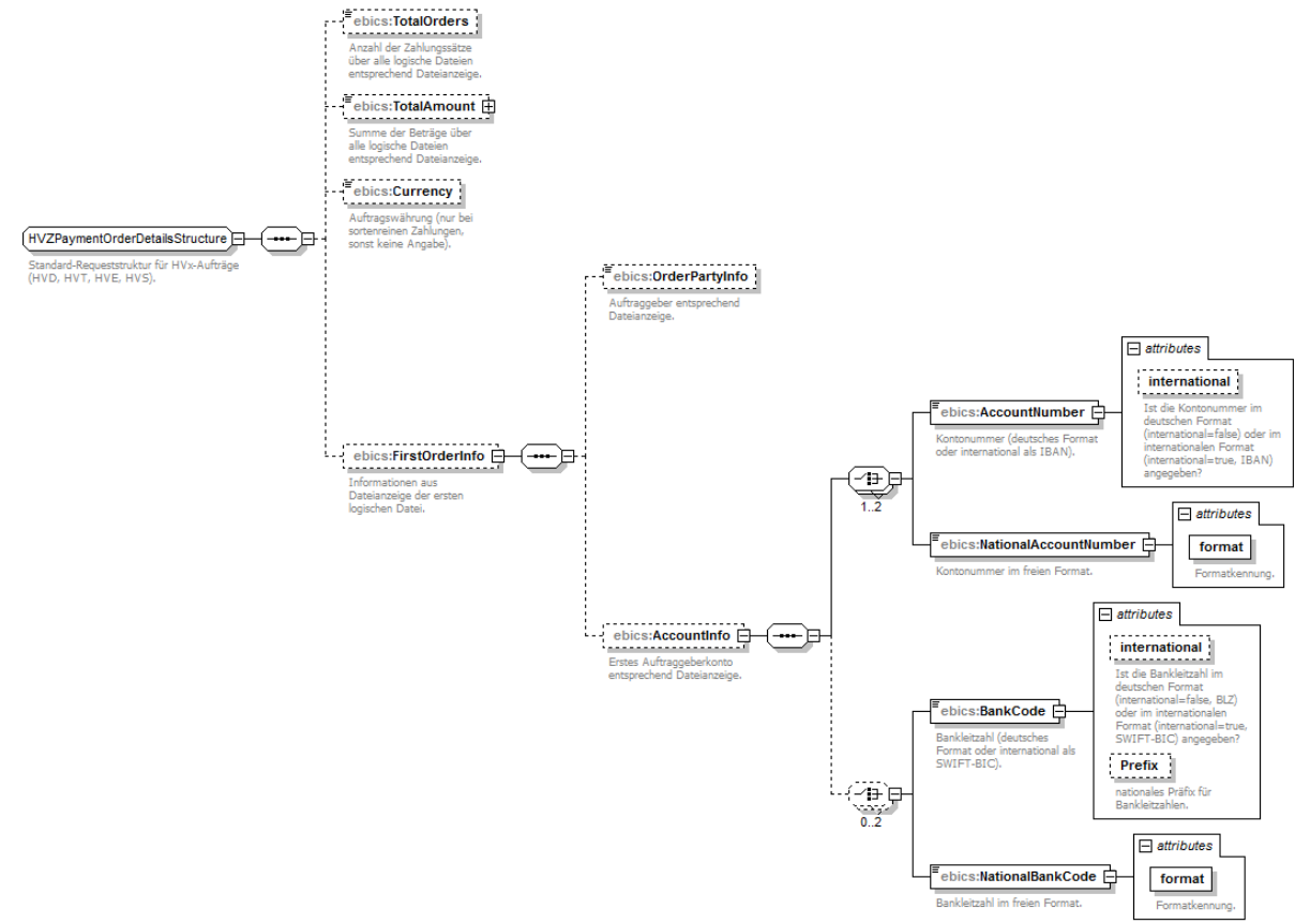
Abbildung 74 HVZPaymentOrderDetailsStructure
