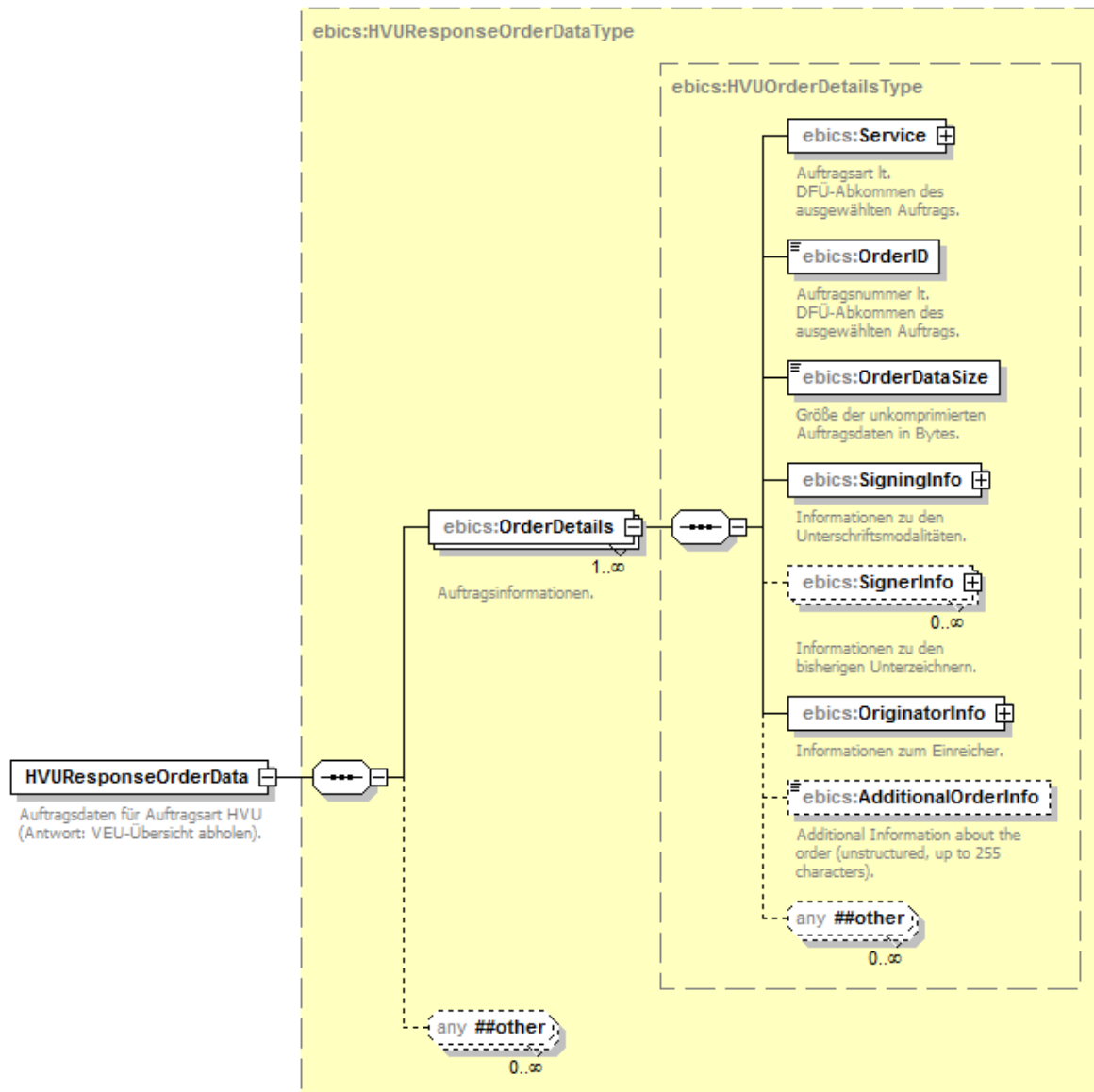
Abbildung 68: HVUResponseOrderData
