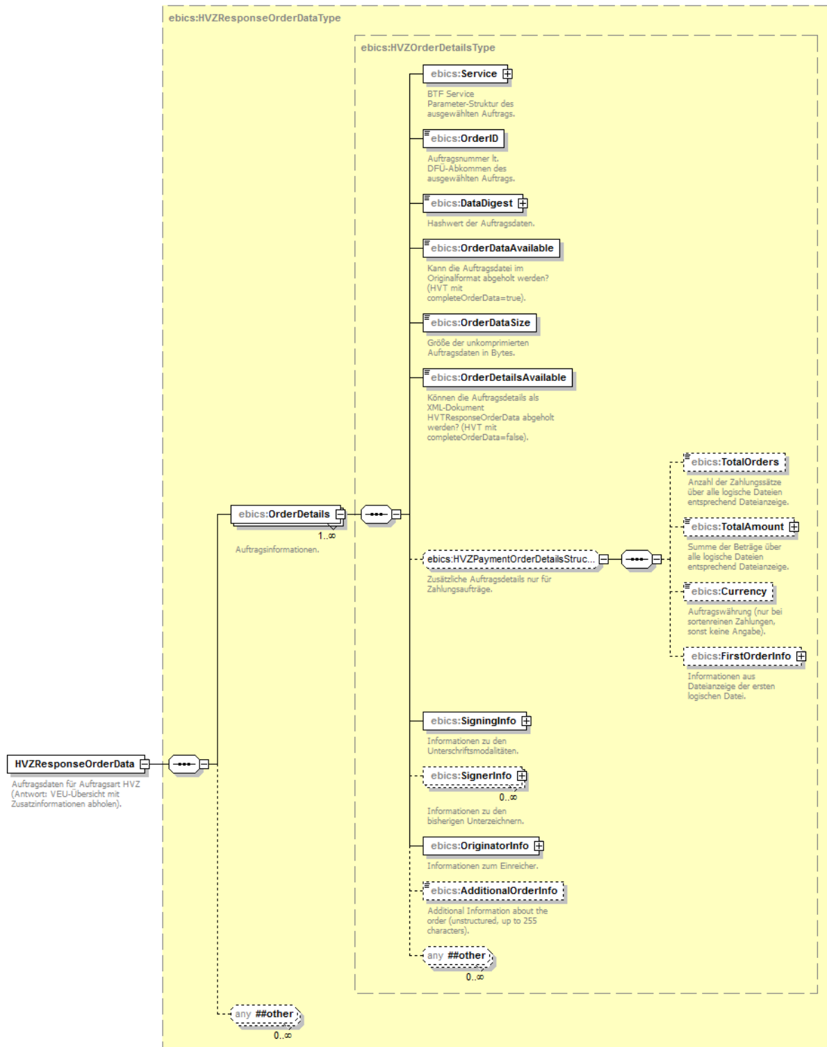
Abbildung 73: HVZResponseOrderData
