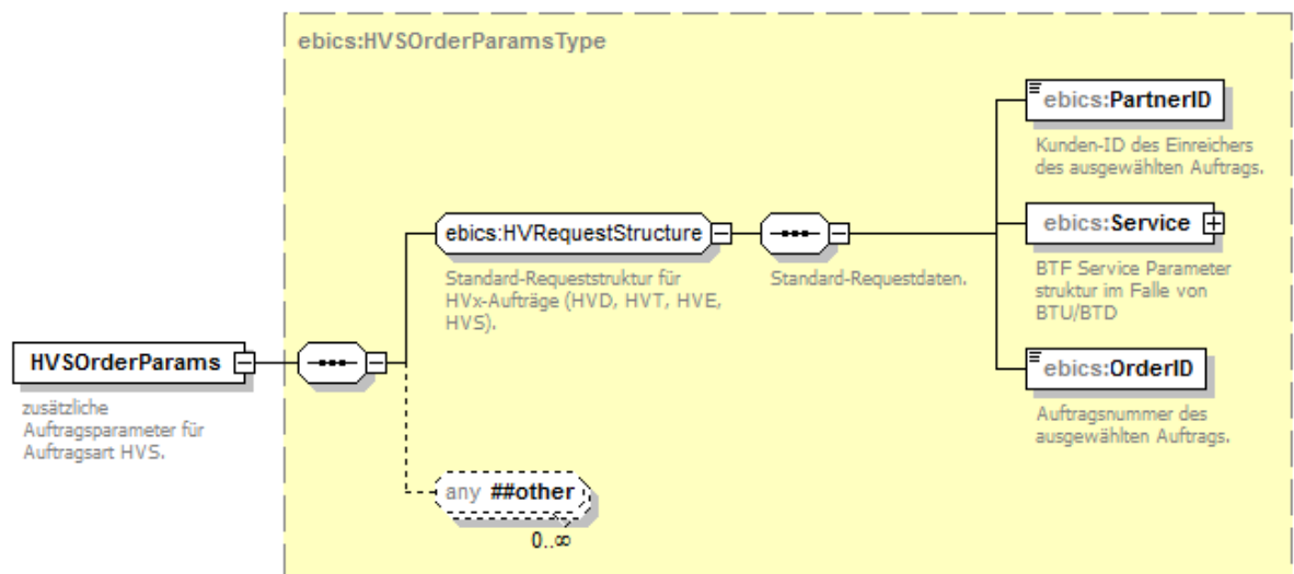
Abbildung 82: HVSOrderParams
