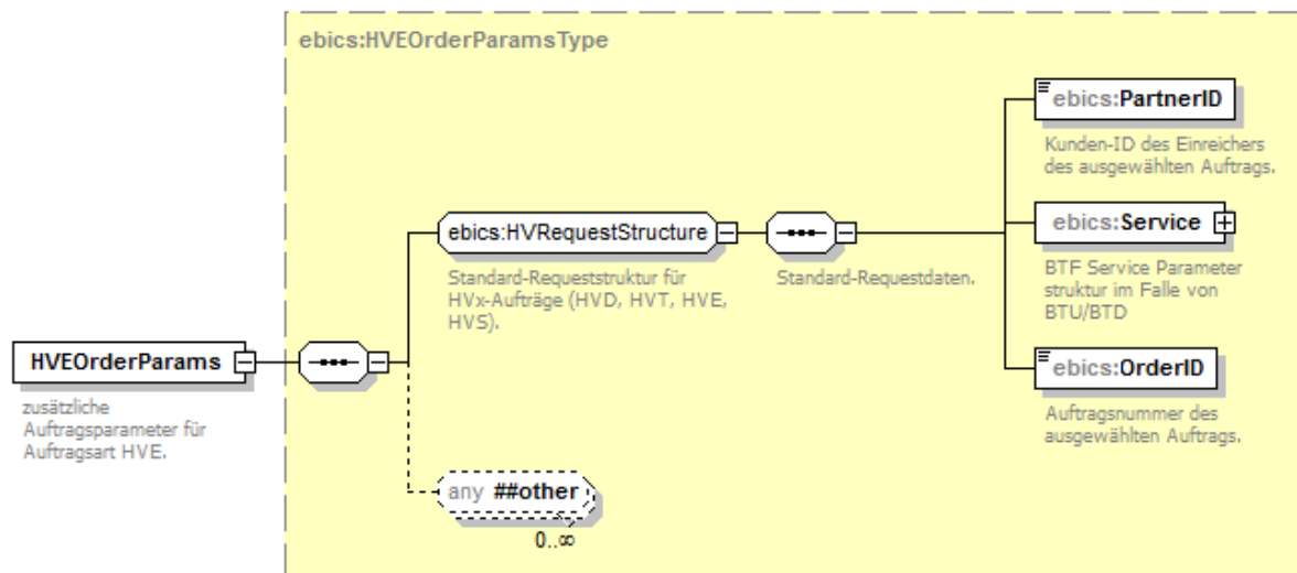
Abbildung 81: HVEOrderParams
