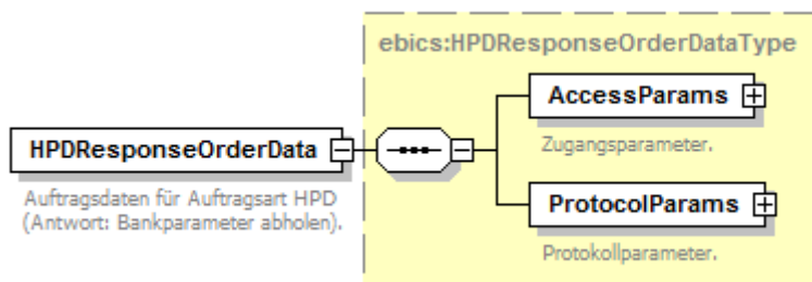
Abbildung 86: HPDResponseOrderData
