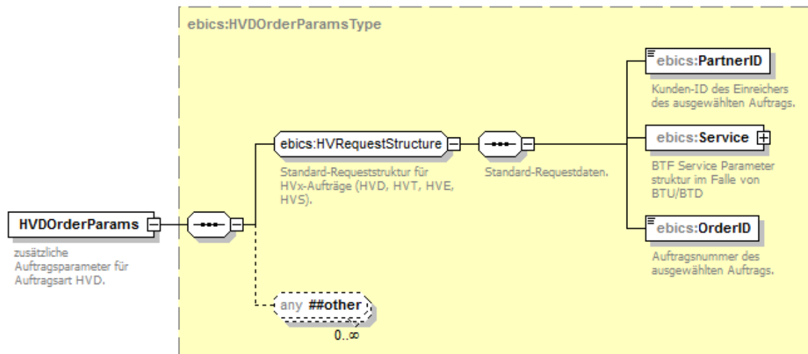
Abbildung 75: HVDOrderParams
