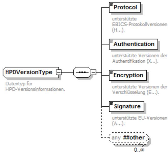
Abbildung 89: HPDVersionType (zu Version)
