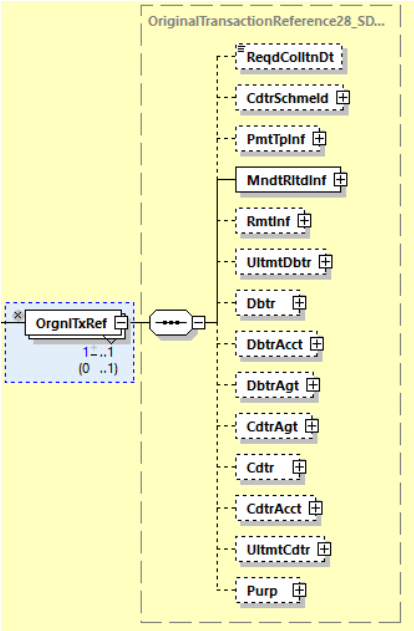
Abbildung 144: Übersicht pain.007.001.09, OrgnlTxRef
