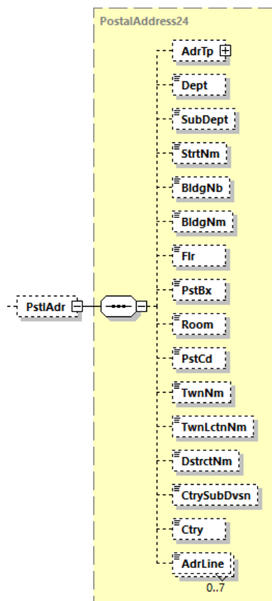
Abbildung 123: camt.053.001.08, PstlAdr
