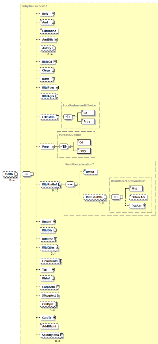
Abbildung 108: camt.053.001.08, TxDtIs
