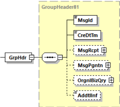
Abbildung 57: camt.054.001.08, GrpHdr
