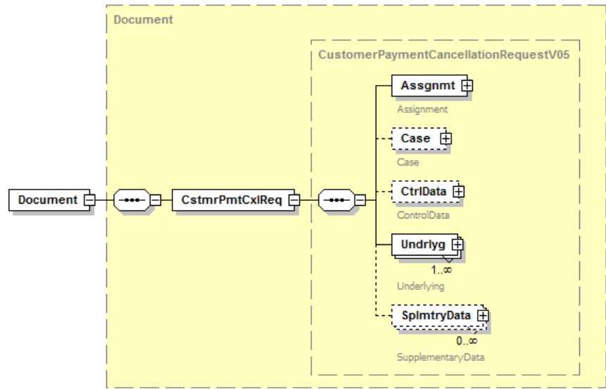
Abbildung 145: Übersicht camt.055.001.05
