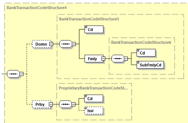
Abbildung 127: camt.053.001.08, BankTransactionCodeStructure4
