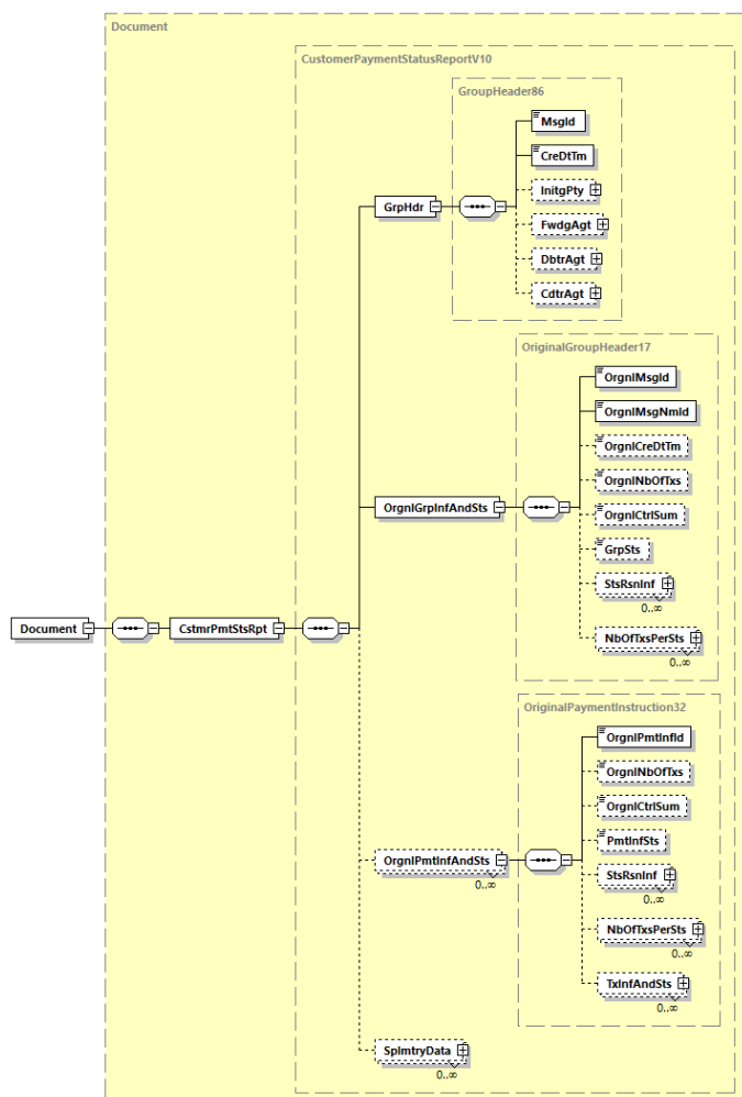
Abbildung 43: Übersicht pain.002.001.10
