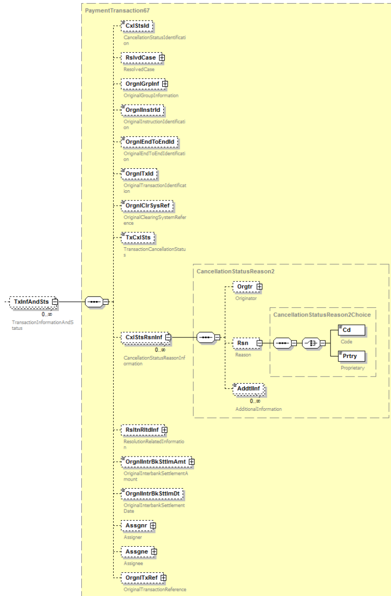
Abbildung 159: camt.029.001.06, TxInfAndSts
