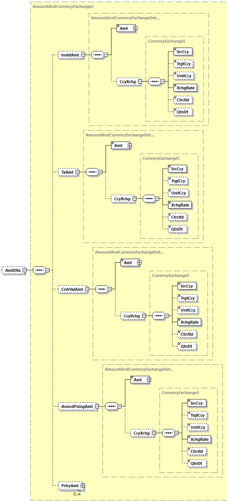
Abbildung 110: camt.053.001.08, AmtDtls
