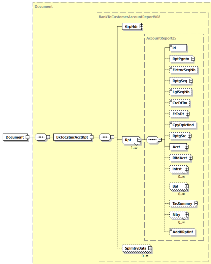
Abbildung 132: Übersicht camt.052.001.08
