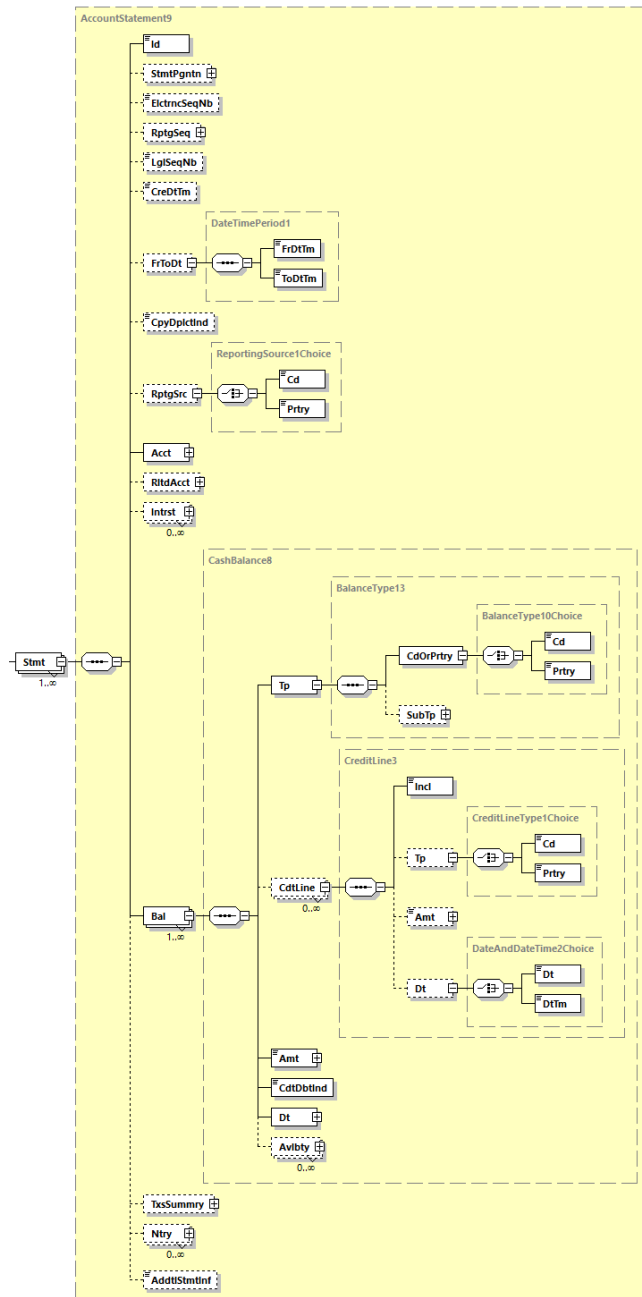
Abbildung 104: camt.053.001.08, Stmnt
