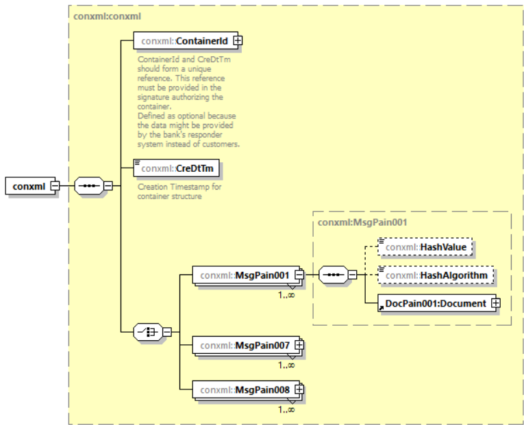
Abbildung 134: Übersicht XML-Container
