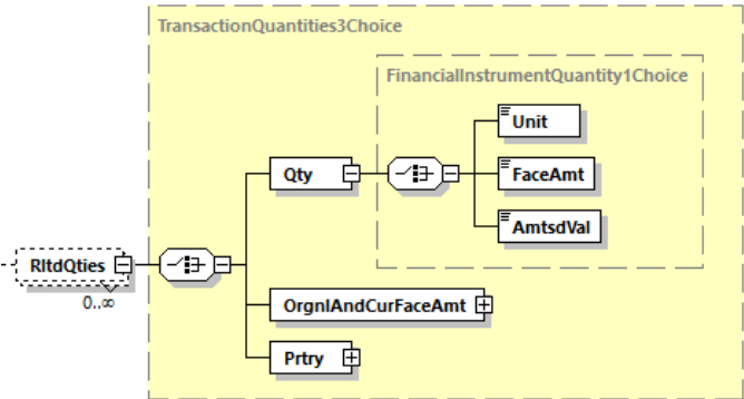
Abbildung 117: camt.053.001.08, RltdQtyes
