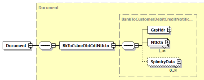
Abbildung 56: camt.054.001.08
