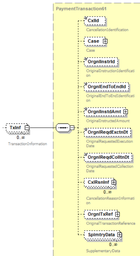
Abbildung 151: camt.055.001.05, TxInf
