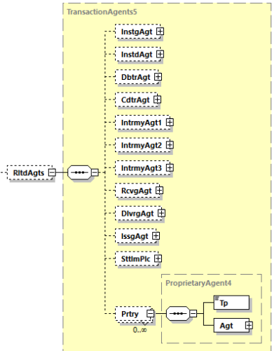
Abbildung 113: camt.053.001.08, RltdAgts
