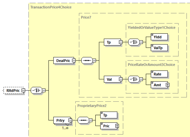
Abbildung 116: camt.053.001.08, RltdPric
