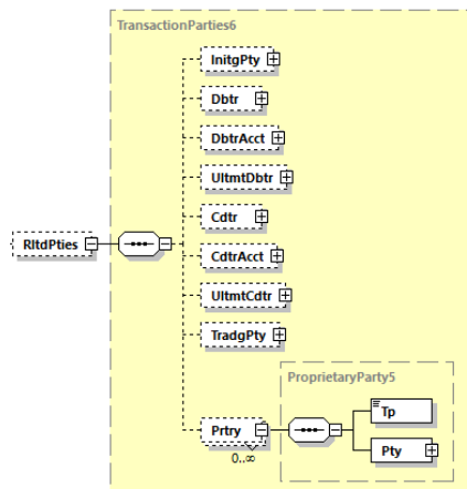
Abbildung 112: camt.053.001.08, RltdPties
