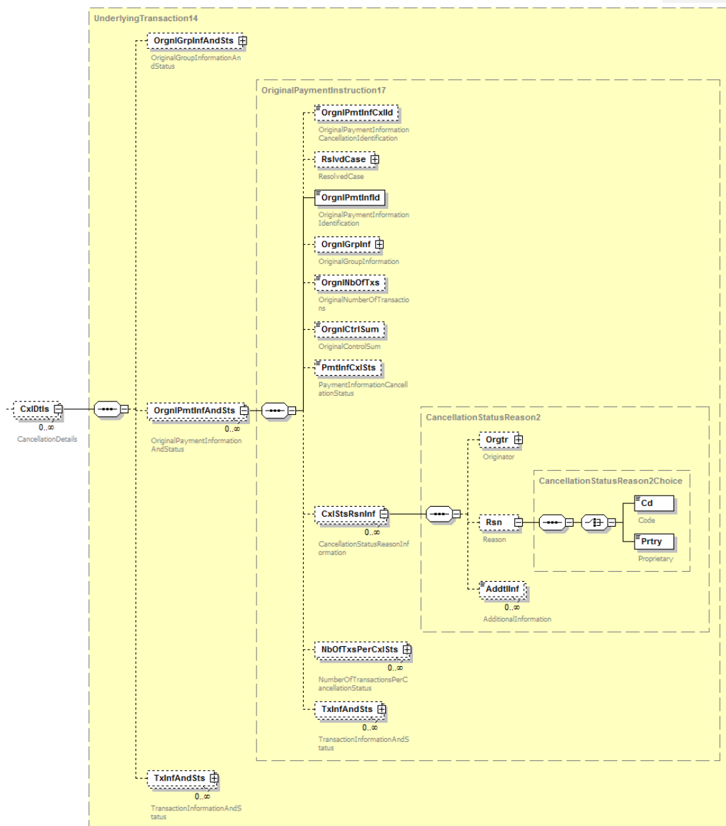
Abbildung 158: camt.029.001.06, CxIDtls
