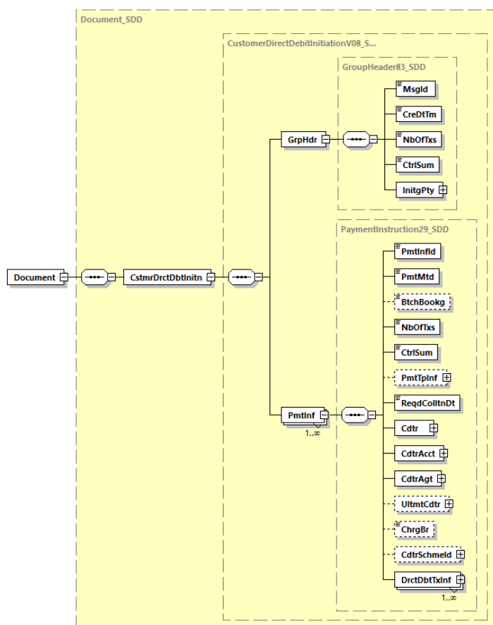
Abbildung 31: Übersicht pain.008.001.08
