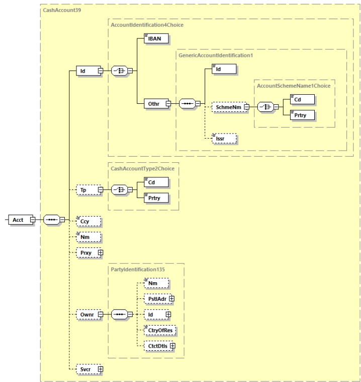
Abbildung 105: camt.053.001.08, Acct
