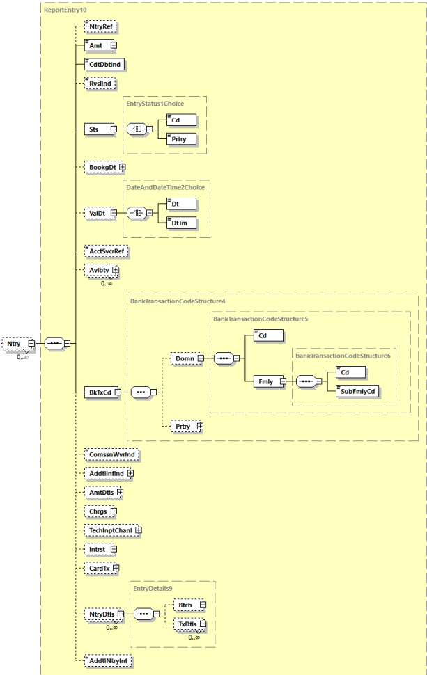
Abbildung 60: camt.054.001.08, Ntry
