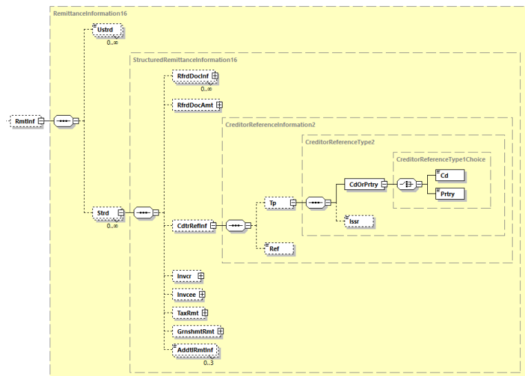
Abbildung 63: camt.054.001.08, RmtInf
