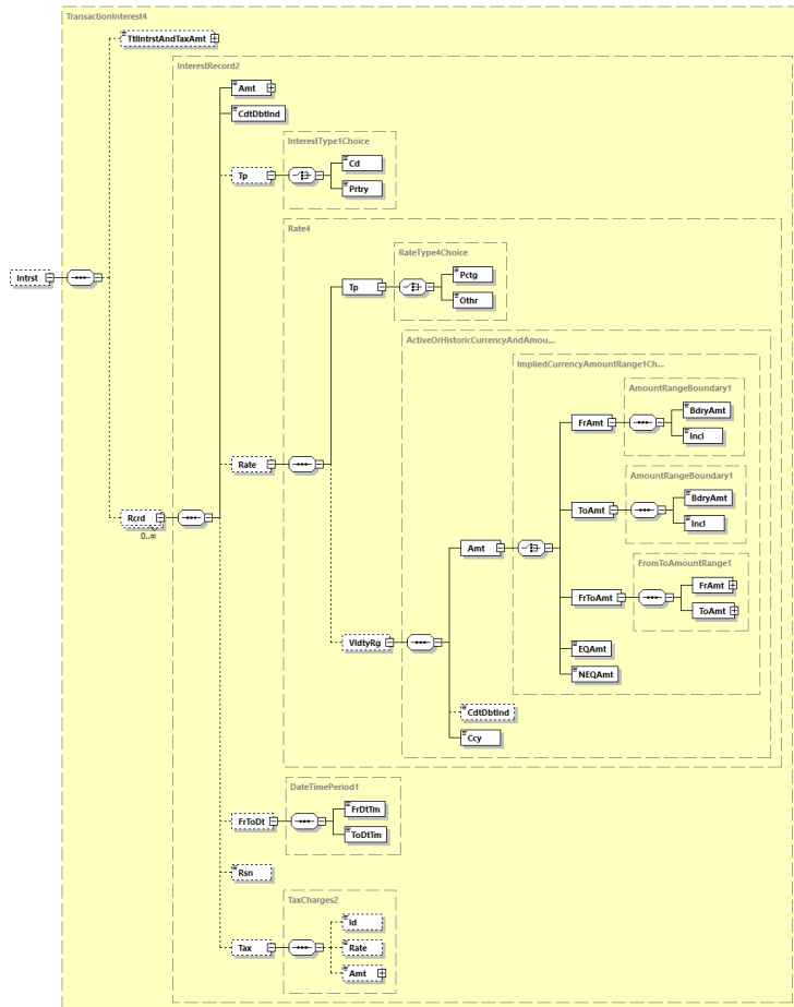
Abbildung 111: camt.053.001.08, Intrst
