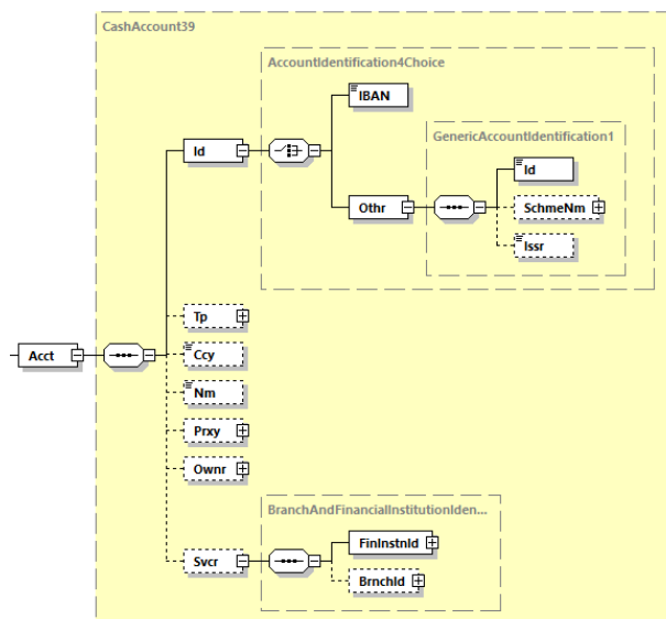
Abbildung 59: camt.054.001.08, Acct
