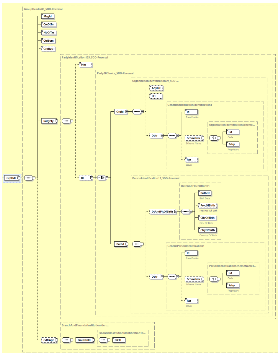
Abbildung 149: Übersicht pain.007.001.09, GrpHdr
