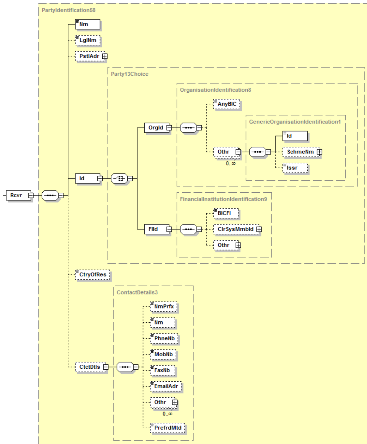
Abbildung 173: Übersicht camt.086.001.02, Rcvr
