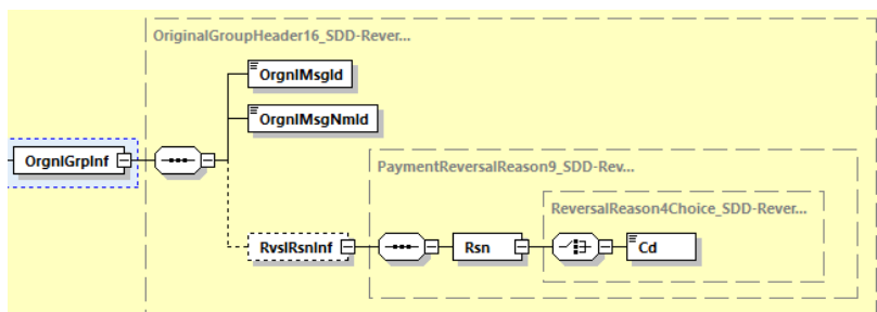
Abbildung 150: Übersicht pain.007.001.09, OrgnlGrplnf
