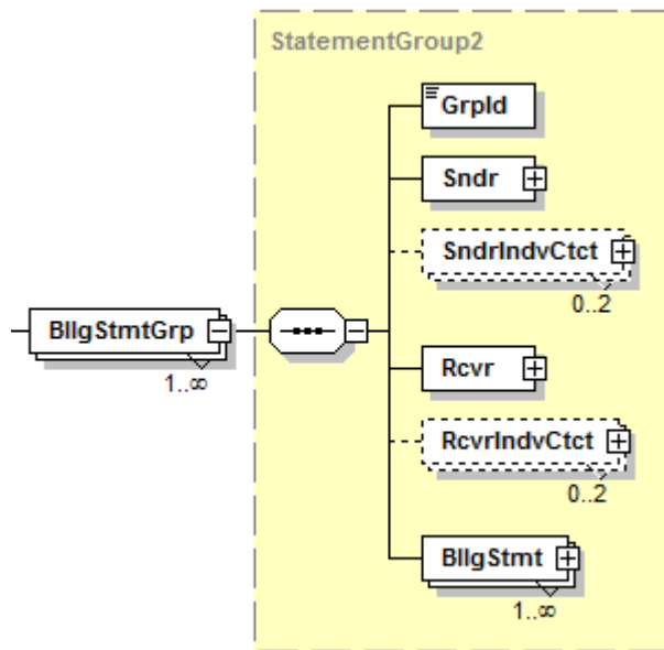
Abbildung 171: Übersicht camt.086.001.02, BllgStmntGrp
