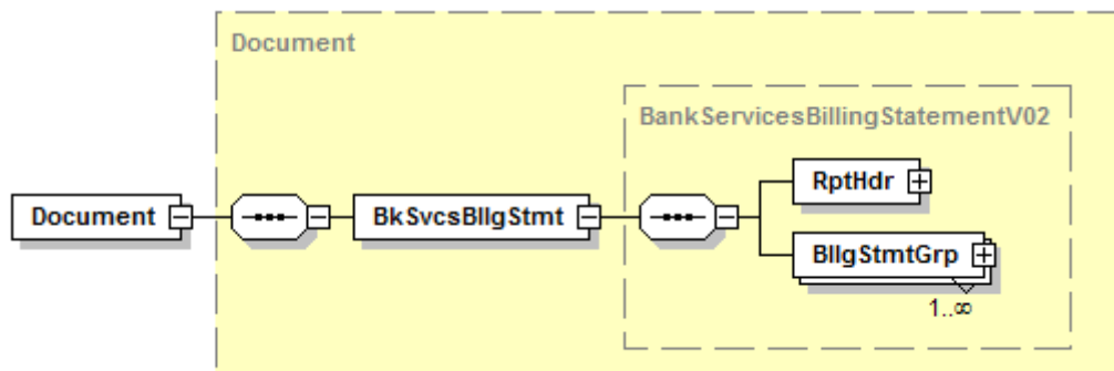
Abbildung 169: Übersicht camt.086.001.02, document
