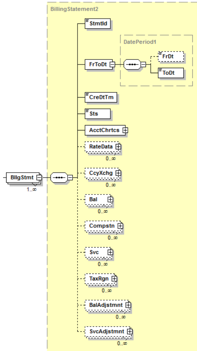
Abbildung 174: Übersicht camt.086.001.02, BlgStmnt
