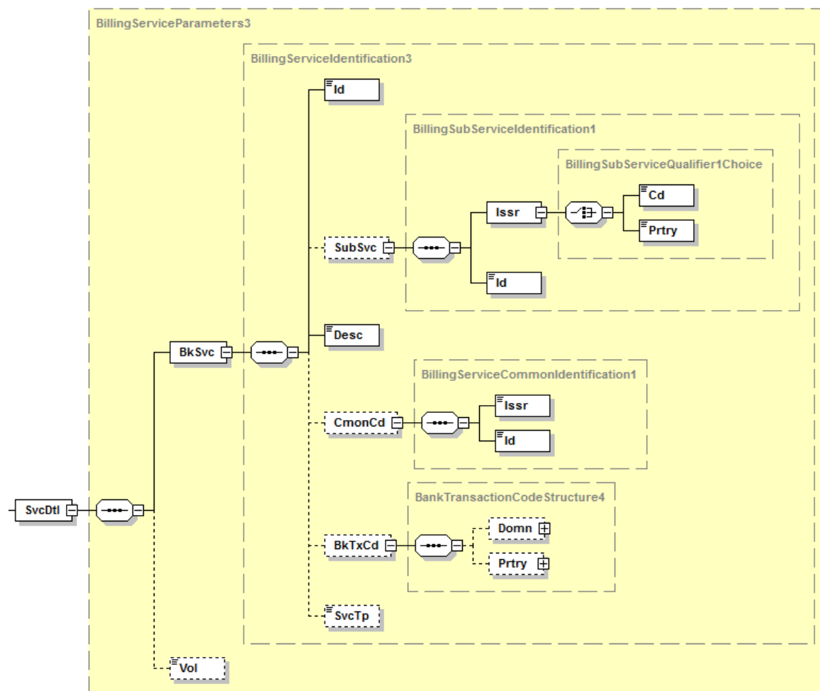
Abbildung 181: Übersicht camt.086.001.02, SvcDtl
