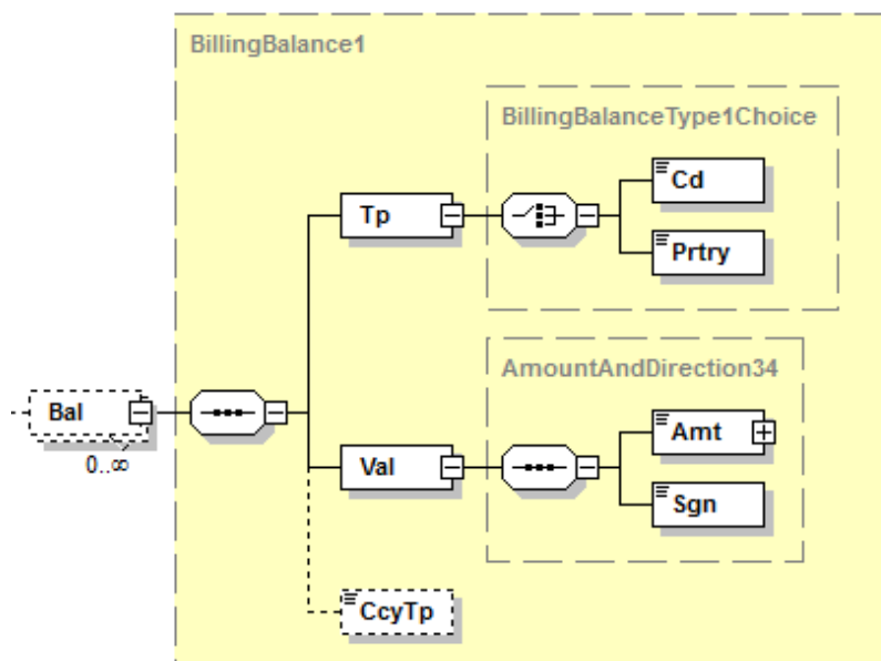
Abbildung 177: Übersicht camt.086.001.02, Bal
