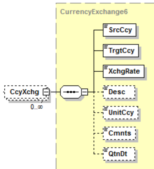
Abbildung 176: Übersicht camt.086.001.02, CcyXchg
