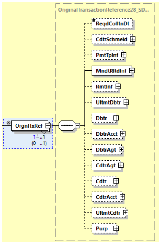
Abbildung 152: Übersicht pain.007.001.09, OrgnlTxRef
