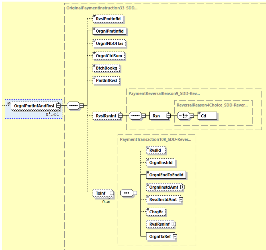
Abbildung 151: Übersicht pain.007.001.09, OrgnPmtInfAndRvsl
