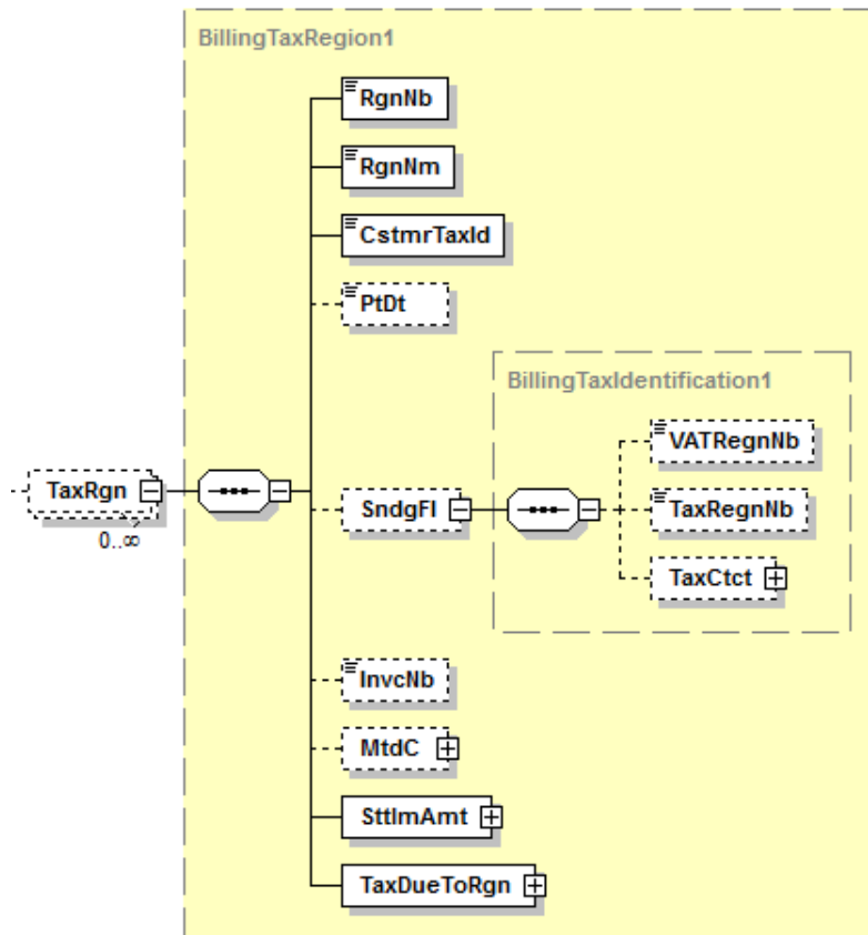
Abbildung 182: Übersicht camt.086.001.02, TaxRgn
