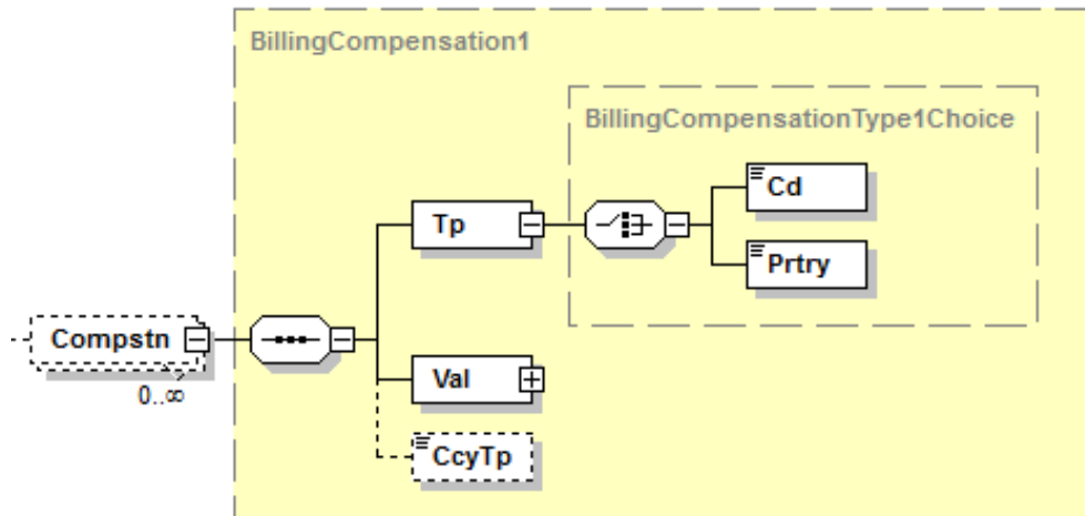
Abbildung 179: Übersicht camt.086.001.02, Compstn
