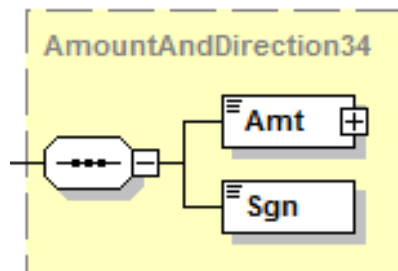
Abbildung 178: Elementstruktur für Darstellung von Beträgen
