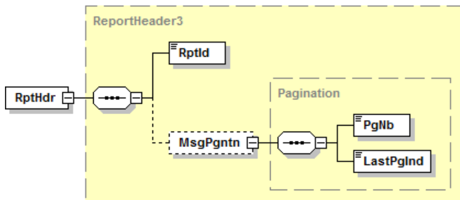
Abbildung 170: Übersicht camt.086.001.02, RptHdr
