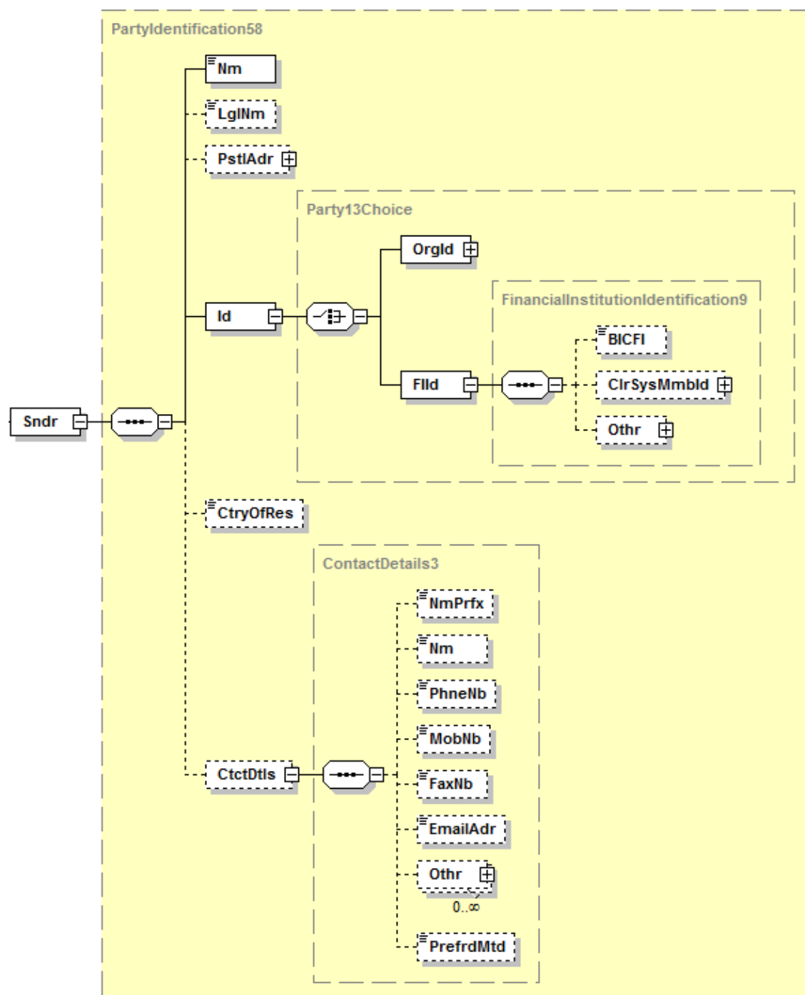
Abbildung 172: Übersicht camt.086.001.02, Sndr
